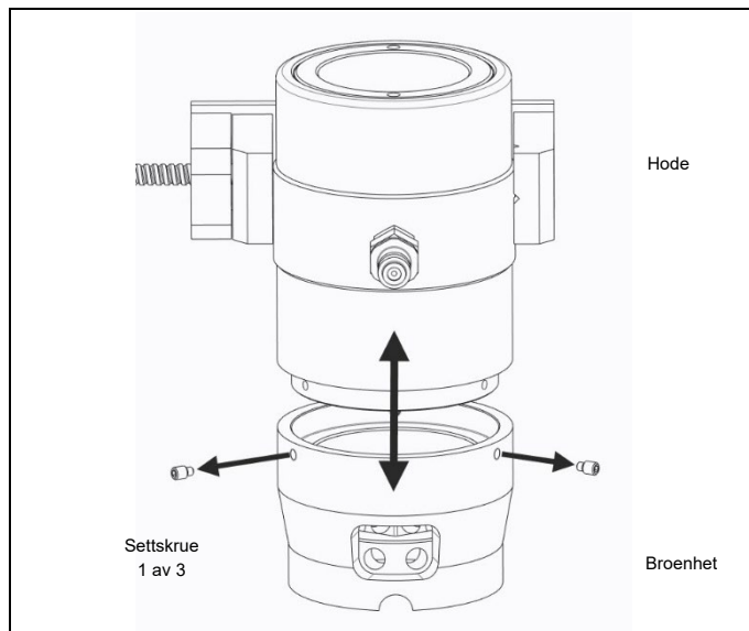
Fig. 4.1 Atskillelse av hode og bro
