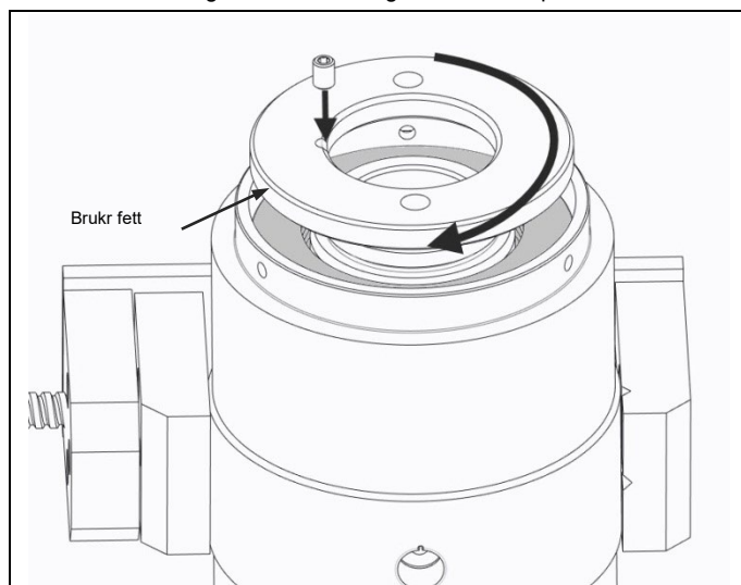
Fig. 4.8 Skru fjærkraven på plass. Sikre med settskrue
