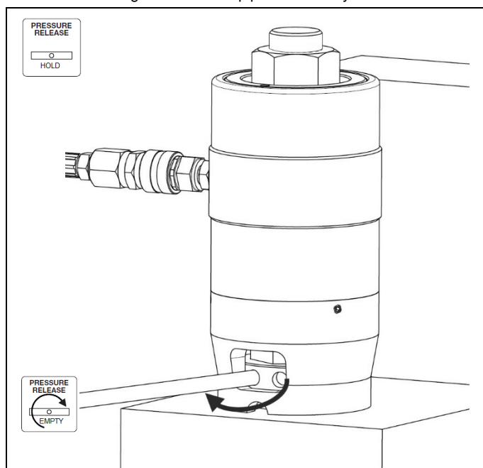
Fig. 2.7 Hold trykket for å stramme mutteren
