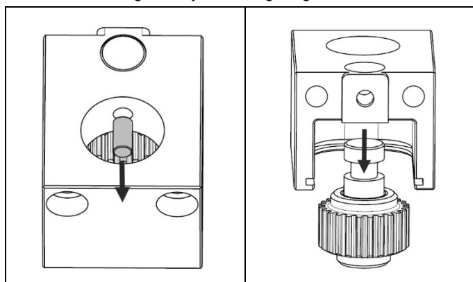
Fig. 4.13 Fjern sikringsstiften etterfulgt av den midterste girenheten
