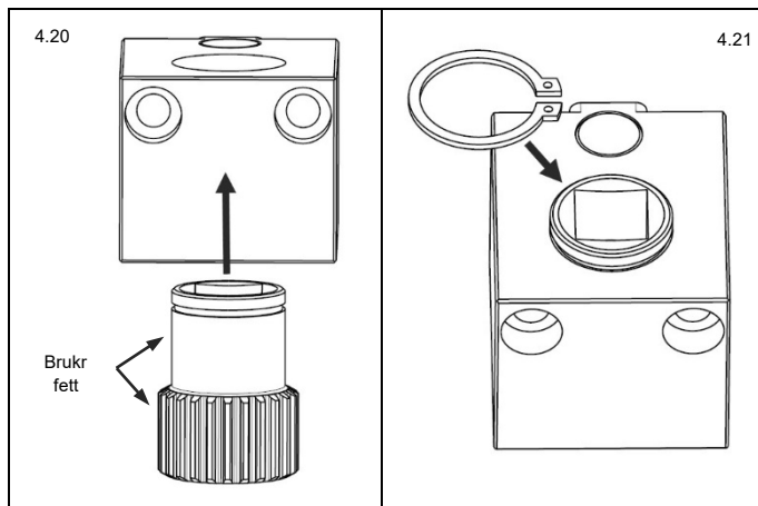
Fig. 4.20 Forbered og installer drevet
