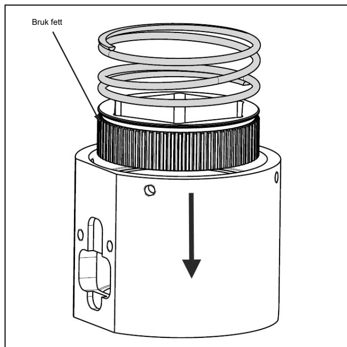
Fig. 4.15 Sjekk at broens indre deler passer riktig, bruk smørefett
