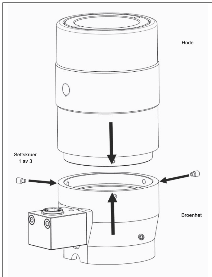
Fig. 4.26 Plasser hodet på broenheten, fest med settskruer
