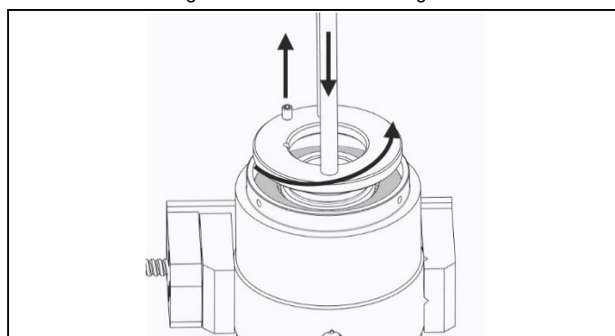
Fig. 4.2 Fjern fjærkraven
