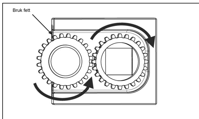
Fig. 4.22 Sjekk at de monterte drevene går jevnt, bruk fett
