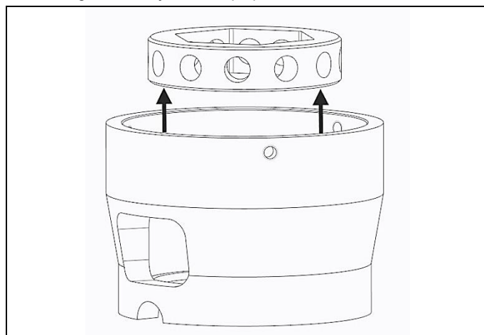
Fig. 4.9 Fjern pipen fra broen
