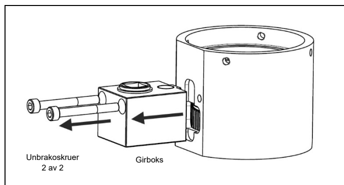
Fig. 4.10 Atskillelse av broenhet og girboks
