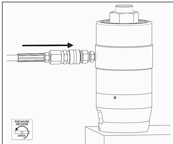
Fig. 2.5 Tilkobling av slange
