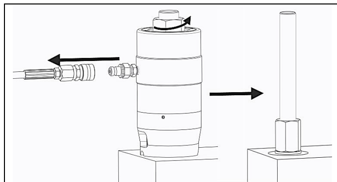
Fig. 2.8 Løsne slangen og flytt strammeren
