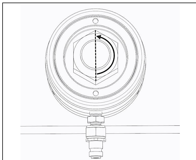
Fig. 3.1 Stram reaksjonsmutteren, og trekk tilbake 1/2 omgang
