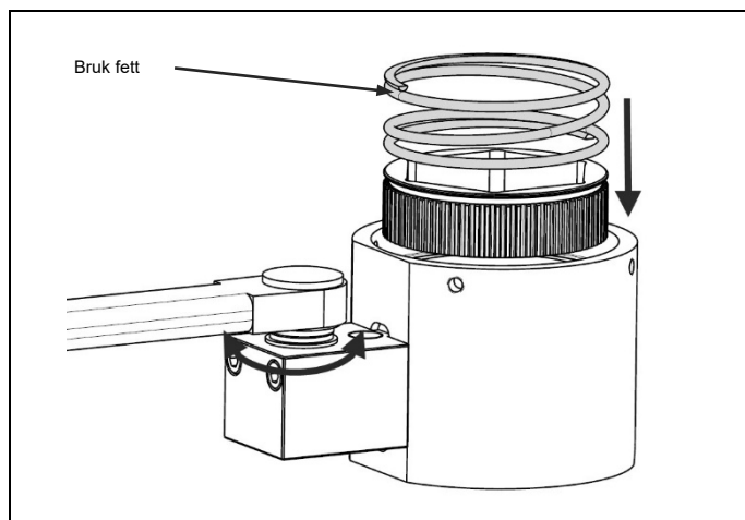
Fig. 4.25 Påfør fett, sett inn tannhylse etterfulgt av fjærer
