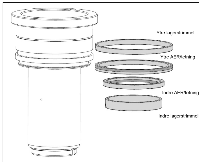
Fig. 4.4 Stempel, ytre AER/tetning, indre AER/tetning, lagerstrimler
