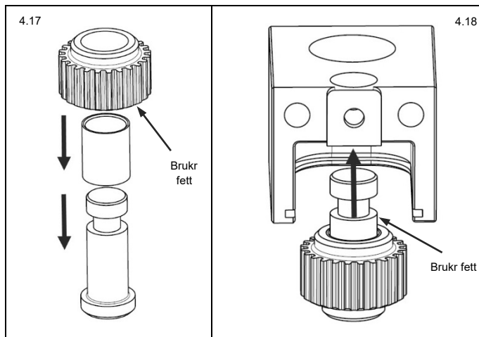
Fig. 4.17 Smør og monter det mellomste drevet
