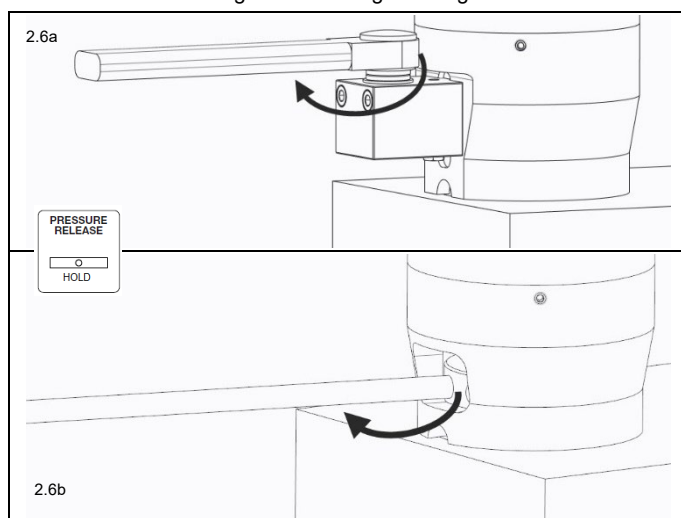
Fig. 2.6a Trekk til pipa med girboksen Fig. 2.6b Trekk til pipa med tommy bar
