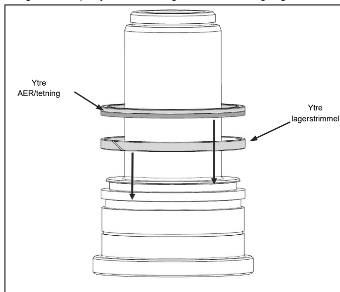
Fig. 4.5 Plasser ytre AER, etterfulgt av ytre tetningen
