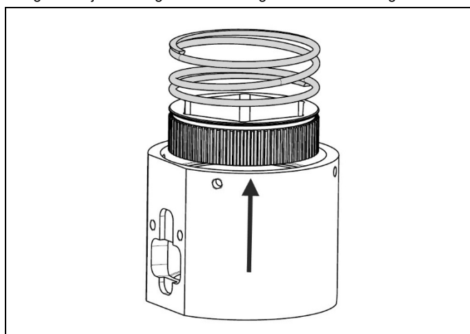
Fig. 4.14 Fjern tannkransen
