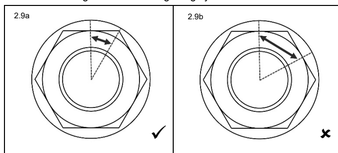
Fig. 2.9a Boltsstramming ferdig
