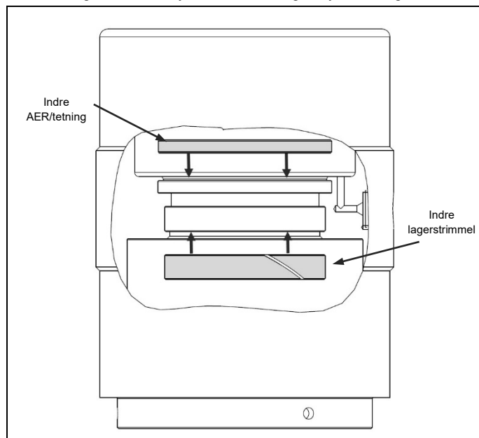
Fig. 4.6 Sett inn indre tetning etterfulgt av den indre AER
