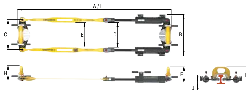
▲ RP70A2L com kit de montagem inferior RP70A2UMK.
