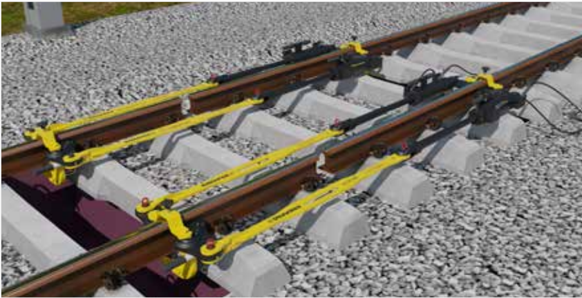
▼ 含 RP70A2L 液压钢轨张拉设备的整套系统。
