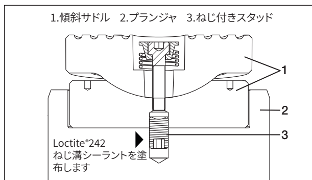
図3: CATSシリーズ傾斜サドルアクセサリ（一般的）
