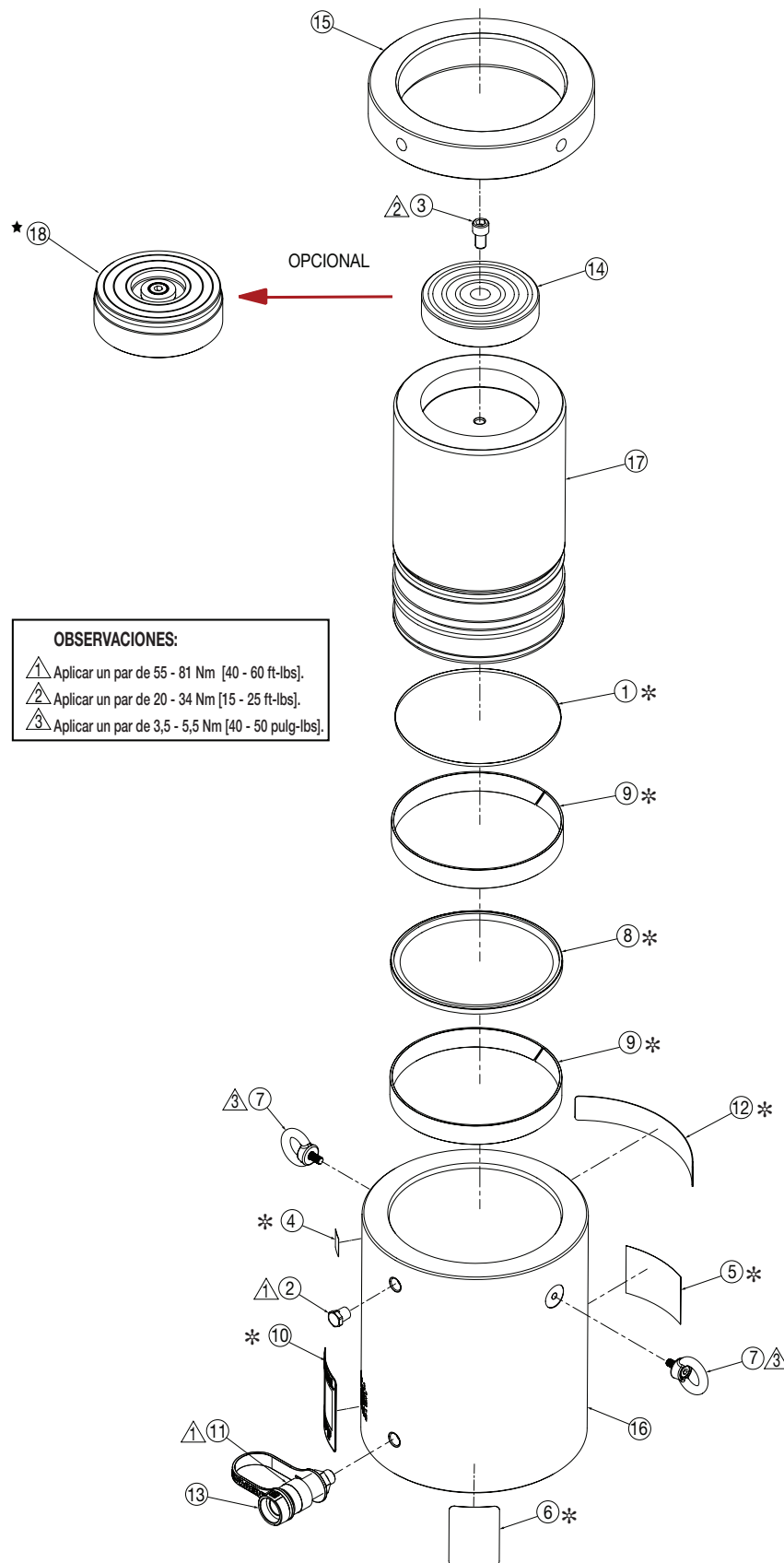
Figura 4, Despiece - Modelo HCL-200
