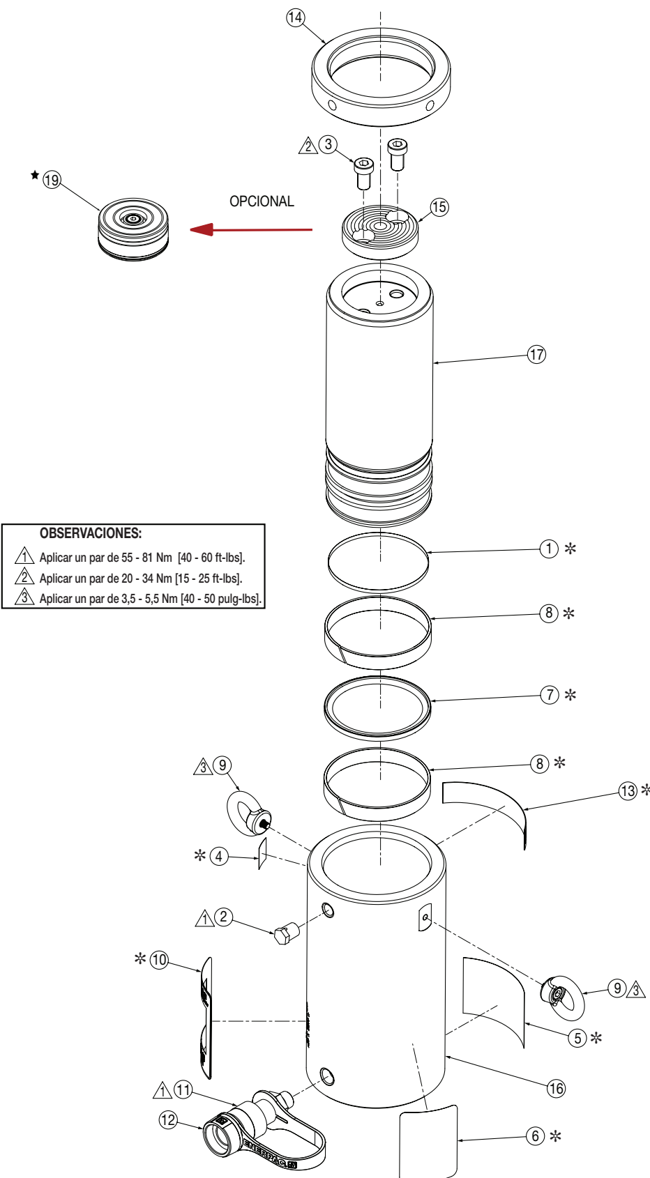
Figura 1, Despiece - Modelo HCL-50
