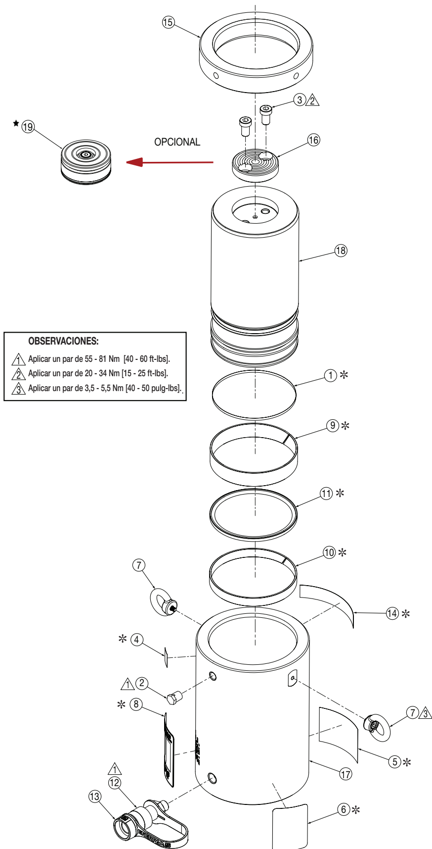
Figura 2, Despiece - Modelo HCL-100
