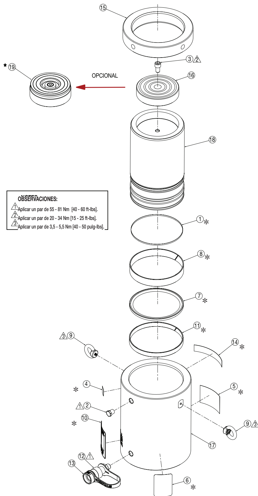
Figura 3, Despiece - Modelo HCL-150
