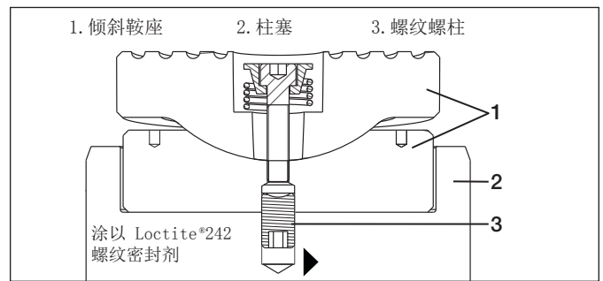
图 4，CATS 系列倾斜鞍座附件（典型）
