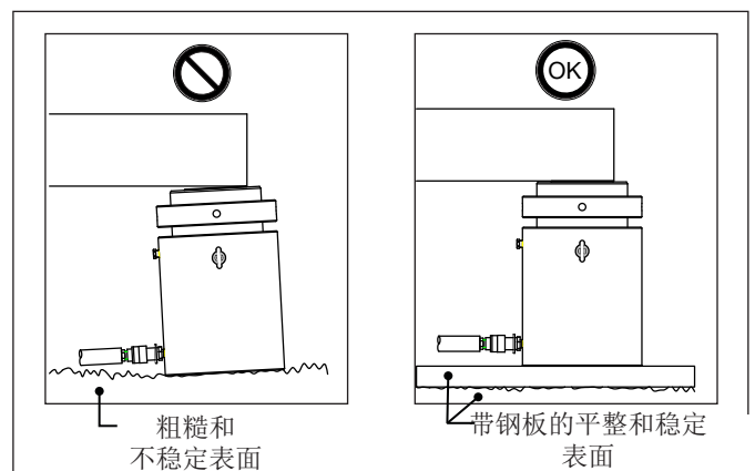
图 5，缸筒支撑
