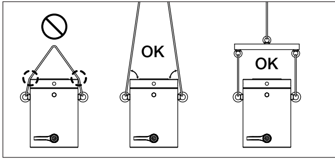
图 3，吊装方法（典型）
