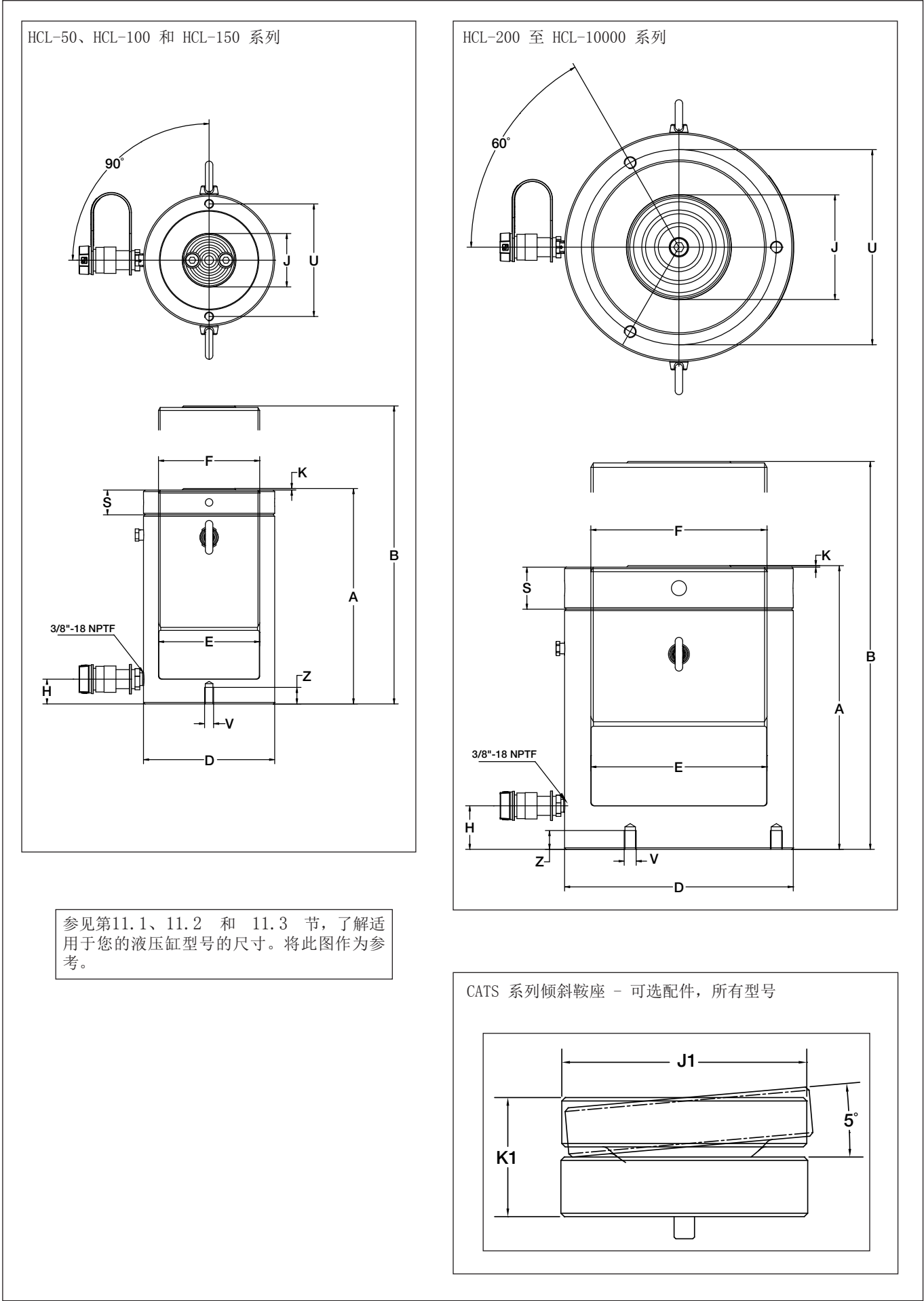
图 7，尺寸 - HCL-系列
