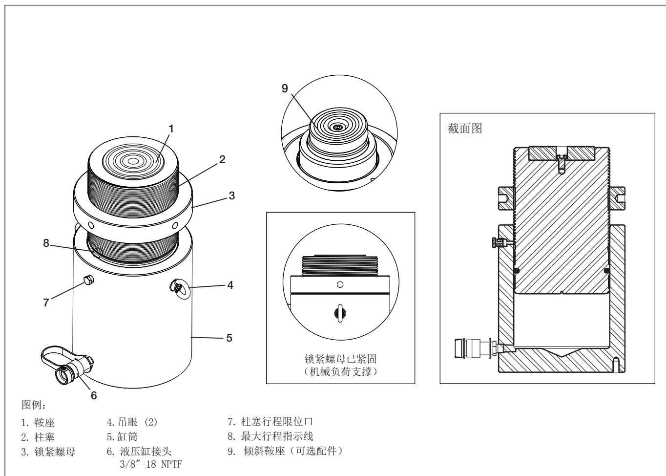
图 2 主要功能和组件
