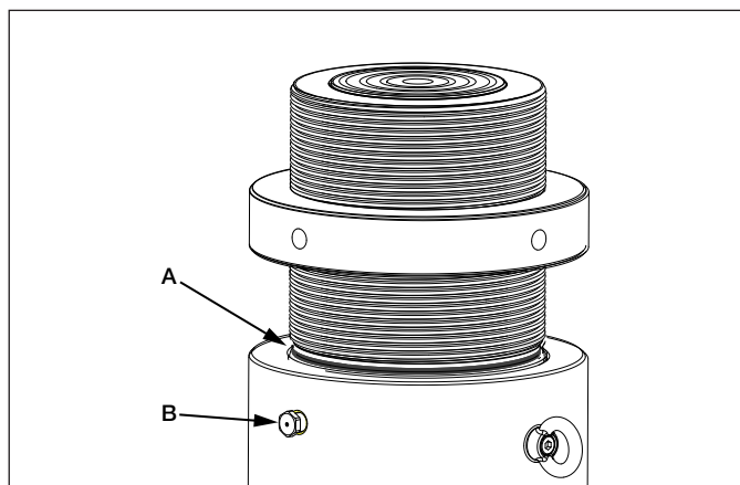
图 6 最大行程指示线 (A) 和柱塞行程限位口 (B)
