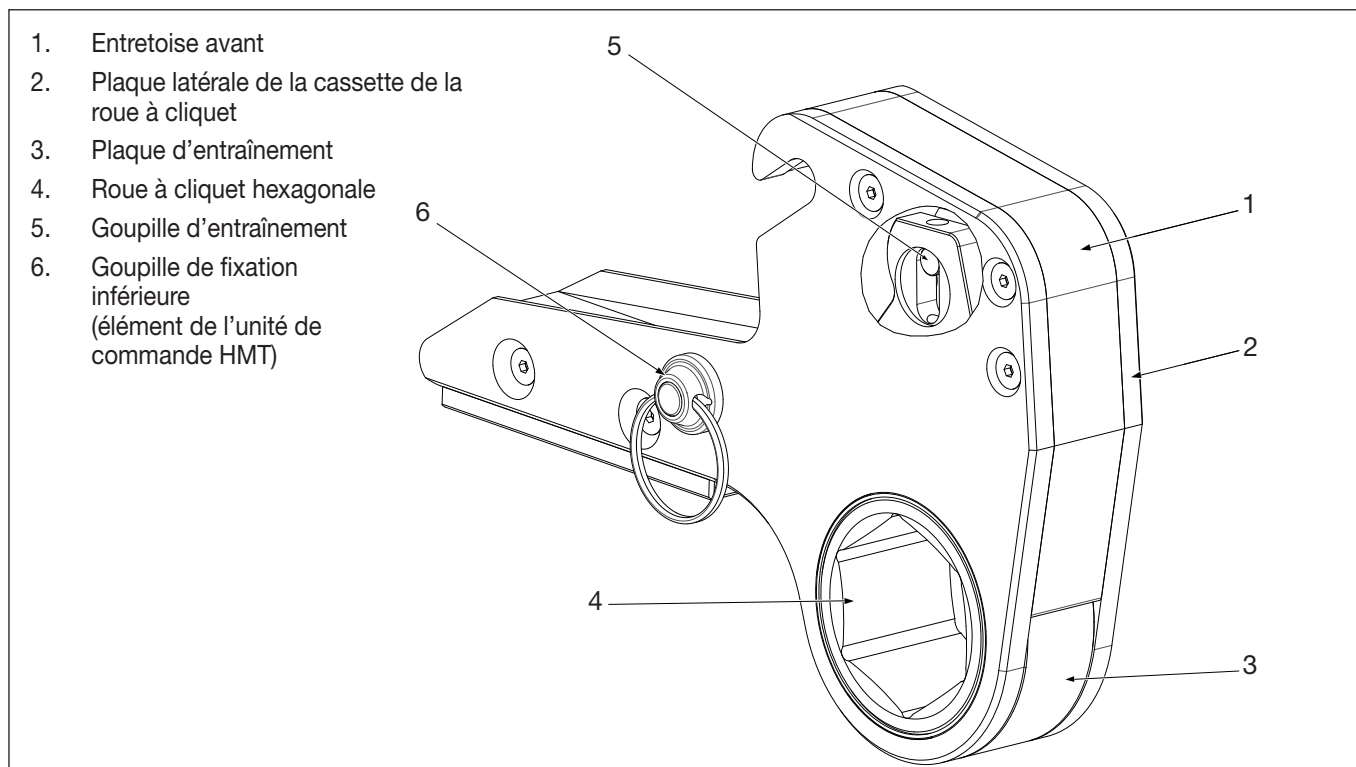
Figure 2 : caractéristiques et composants principaux de la cassette ultra plate HLP HMT
