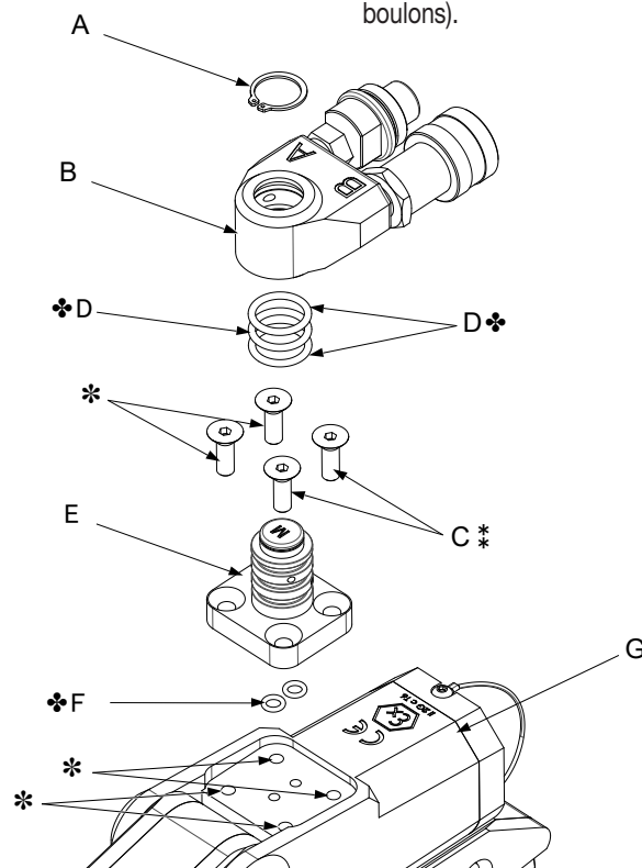
Figure 17 : potelet de raccord tournant et montage du raccord tournant
