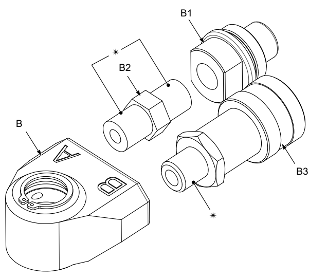
Figure 18 : vue éclatée du montage du raccord tournant
