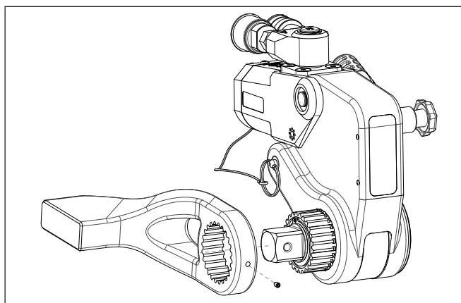
Figure 8 : installation du bras de réaction du carré conducteur
