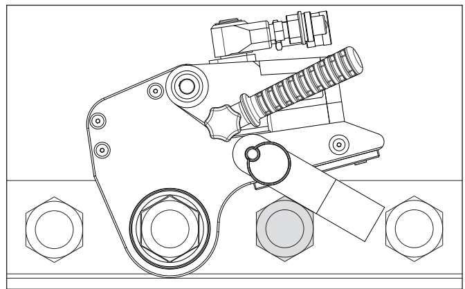
図14: 反力パドルを使用
