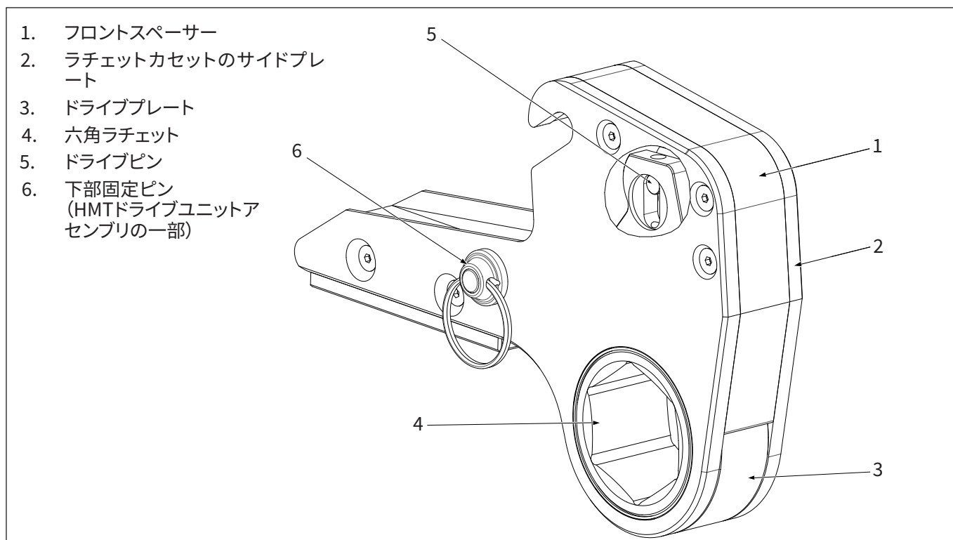
図2: HMT HLP薄型カセットの主な特長と構成部品
