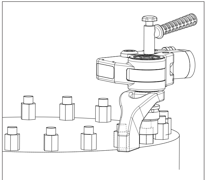
図16: HSQカセットを装着したHMTを適切な反力点に配置
