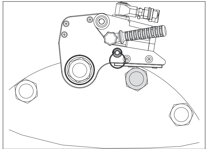
図13: HLPカセットを装着したHMTを適切な反力点に配置
