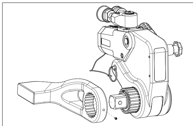
図8: 四角ドライブ反力アームの取り付け
