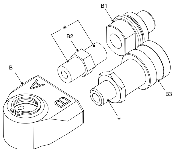
図18: スィベルアッセンブリの展開図
