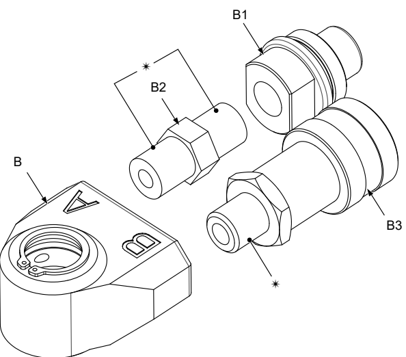
Abbildung 18: Explosionsansicht der Schwenkkupplung
