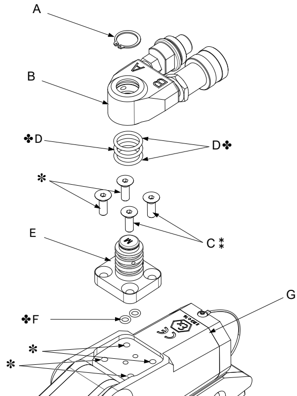
Abbildung 17: Schwenkkupplungsstange und Schwenkkupplung
