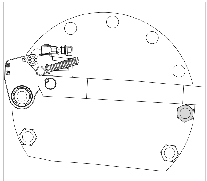
Figuur 15: Gebruik van de verlengde reactiearm
