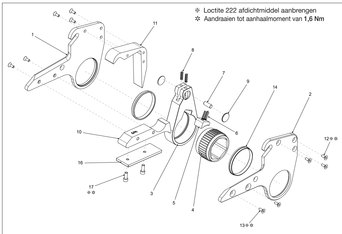
Figuur 20: Opengewerkte tekening van HLP-cassette
