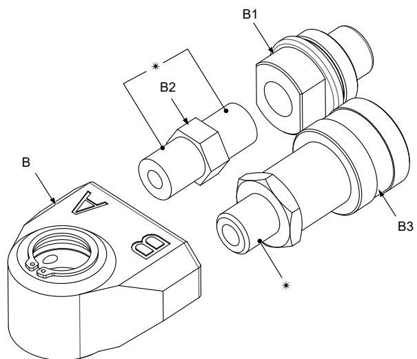
Figuur 18: Opengewerkte tekening van koppelingssset
