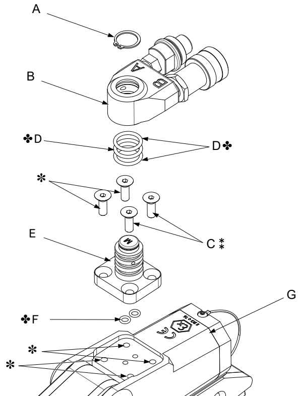
Figuur 17: Koppelingsstang en koppelingssset
