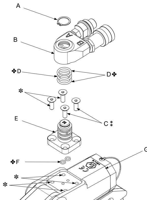
Figura 17: Batente da Conexão Giratória e Conjunto Giratório
