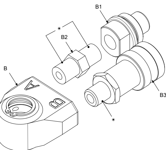
Figura 18: Conjunto Giratório Ampliado
