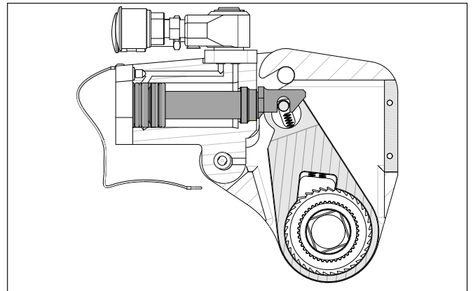
Figura 5: Conexão do Cabeçote HSQ e Unidade de Acionamento da HMT
