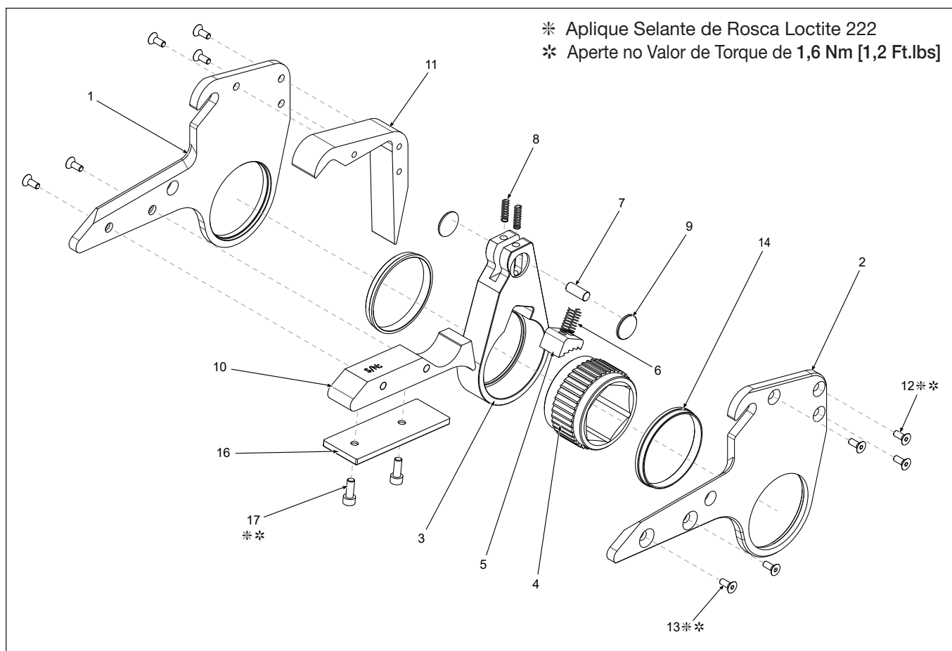
Figura 20: Cabeçote HMT HLP Ampliado
