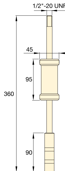
Dimensões do martelo deslizante (mm)
