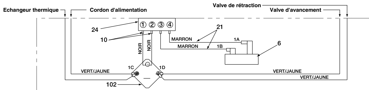
Figure 8, Schéma de câblage
