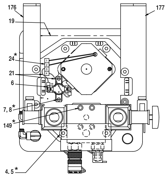
Figure 7, Vue de dessus de la pompe
