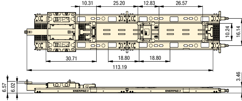
Sistema de deslizamiento de poca altura (dimensiones en pulgadas)
