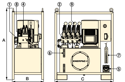
Serie SFP con depósito de 40 galones (mostrado aquí con 4 salidas de flujo dividido)
