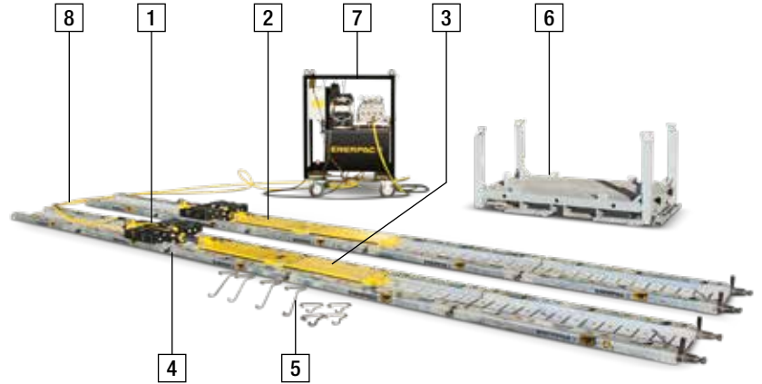
Sistema de deslizamiento de poca altura (dimensiones en pulgadas)
