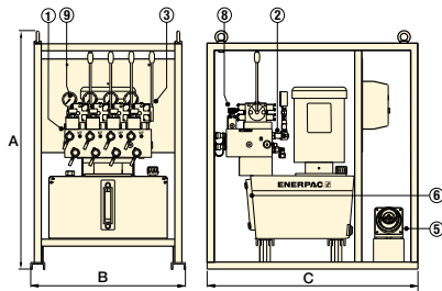
Serie SFP con depósito de 10 galones (mostrado aquí con 4 salidas de flujo dividido)
