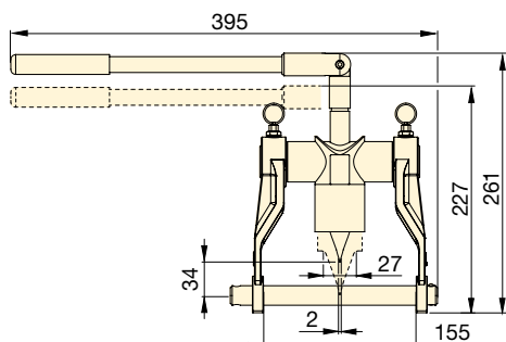
Attrezzo retratto ed esteso con barra di apertura grande (Ø 20 mm)
