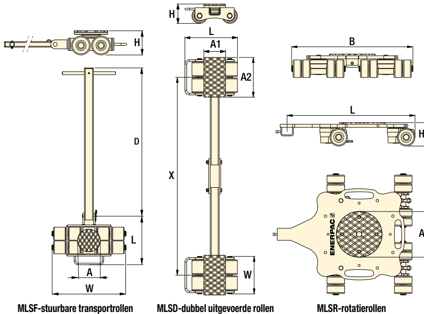
MLSF-stuurbare transportrollen
