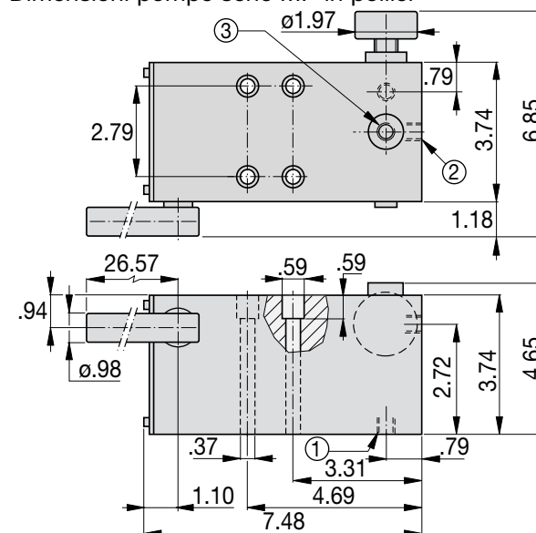
Dimensioni pompe serie MP in pollici
