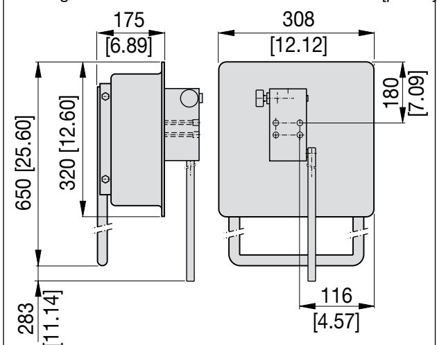
Montage du réservoir MP-10T dimensions en mm [pouce]
