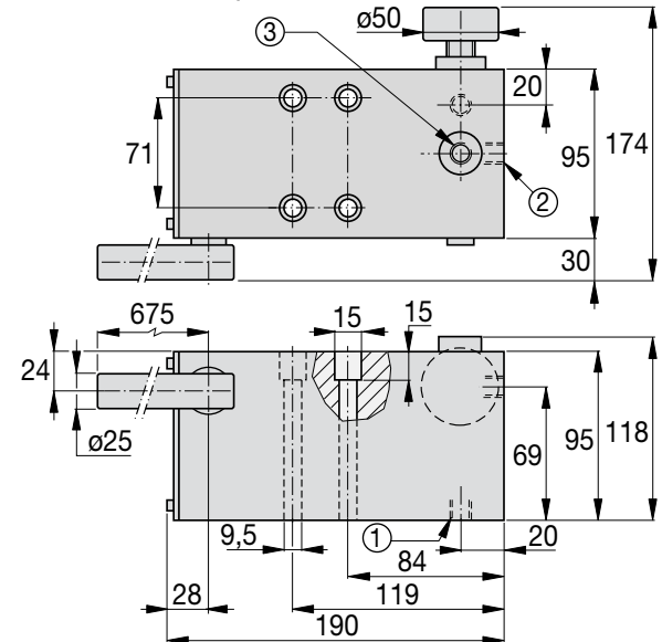
MP-Seriens Pumpdimensioner i millimeter
