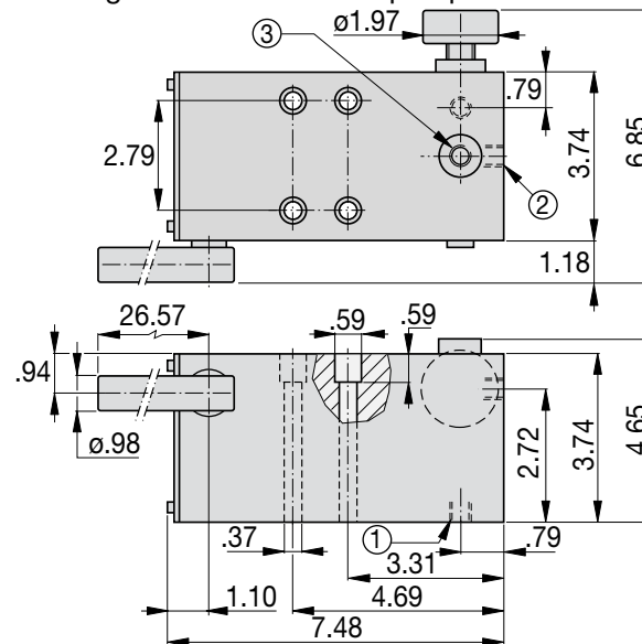
Afmetingen van de MP-serie pomp in inches
