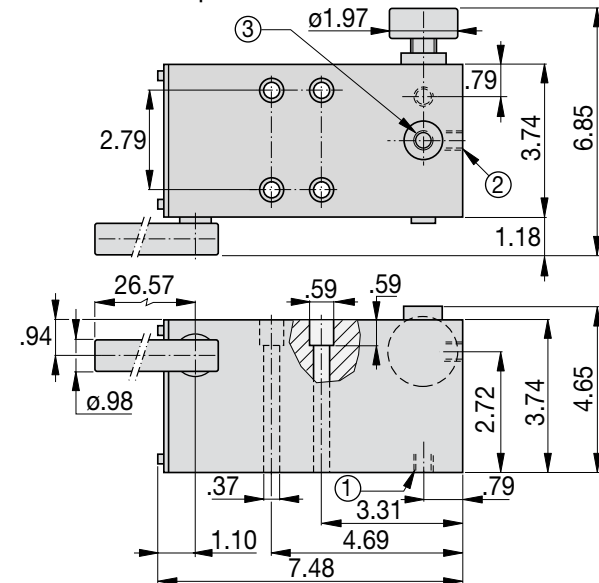
MP-Series Pumpdimensioner i tum
