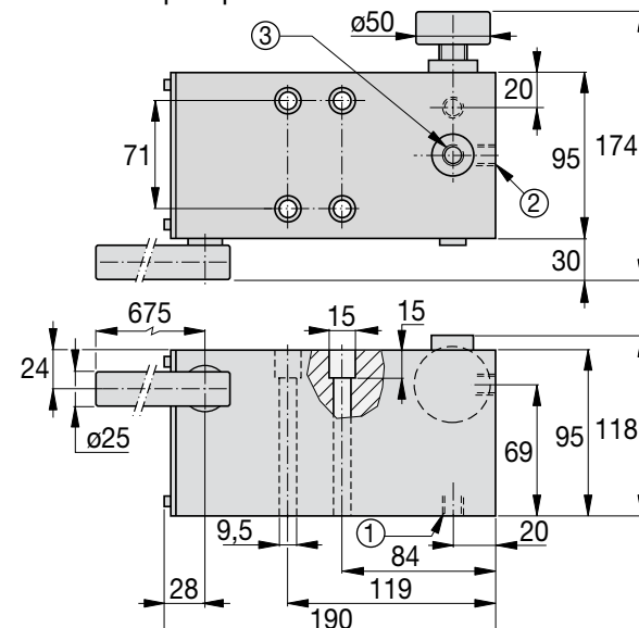
Dimensioni pompe serie MP in millimetri
