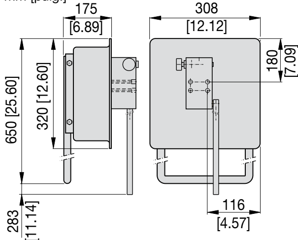
Dimensiones de montaje del depósito MP-10T en mm [pulg.]
