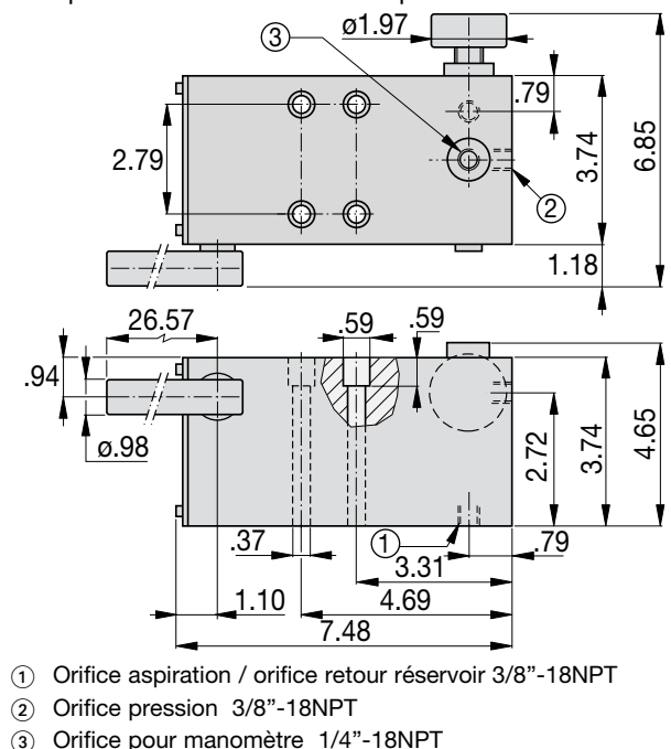
Pompe série MP dimensions en pouces
