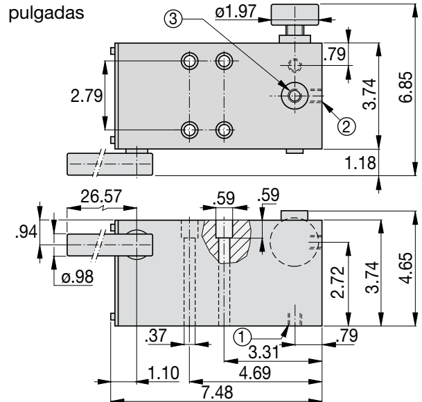
Dimensiones de montaje del depósito MP-10T en mm [pulg.]
