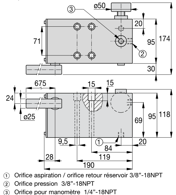
Pompe série MP dimensions en mm
