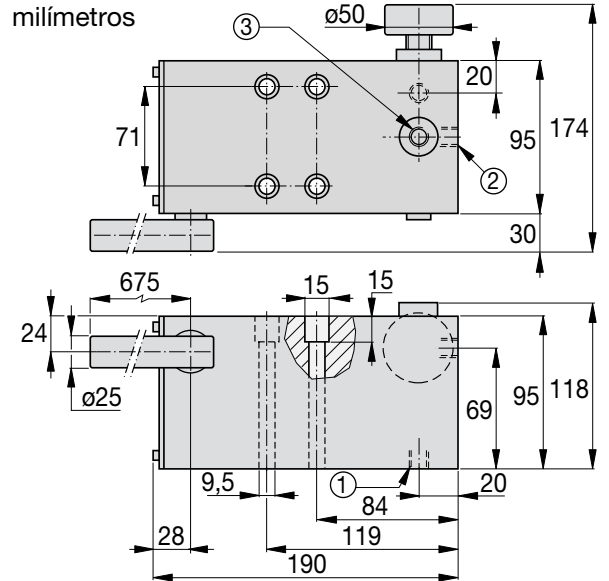
Dimensiones de la bomba de la serie MP en milímetros
