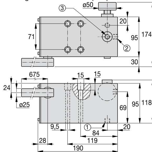
Afmetingen van de MP-serie pomp in millimeters
