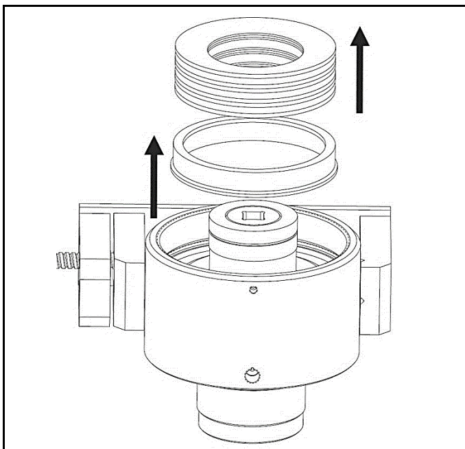
図 4.3 皿バネとスプリングインサートの取り外し
