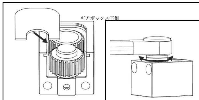
図 4.24 ギアボックスカバーの取り付け、ギアがスムーズに回転するかどうかの点検
