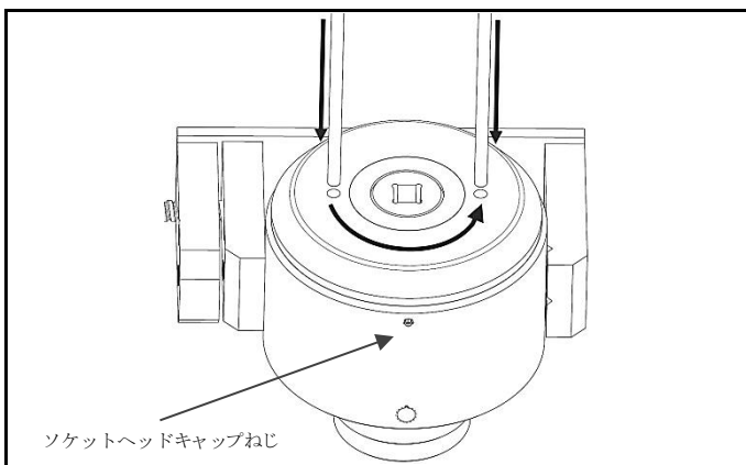
図 4.2 回り柄を使用したスプリングキャップの取り外し
