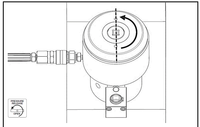
図 3.1 プーラーバーの 1 回転の 3/4 戻した締め付け
