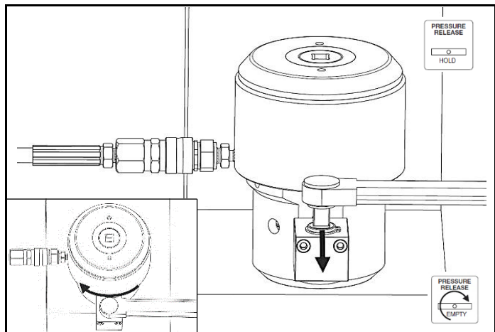
図 2.7 ギアボックスドライブを回してのナットの締め付け
