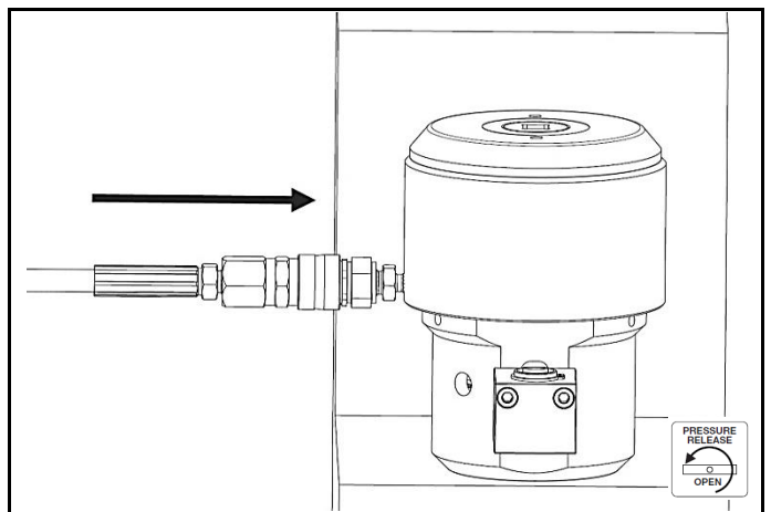
図 2.6 ホースの接続
