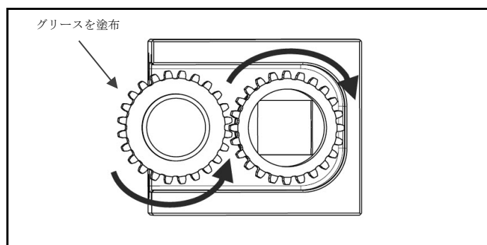
図 4.23 取り付けたギアがスムーズに回転するかどうかの点検、グリースの塗布
