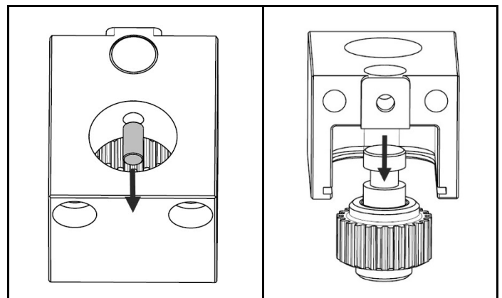
図 4.14 中間ギアアッセンブリの取り外しの後、固定ダウエルピンの取り外し
