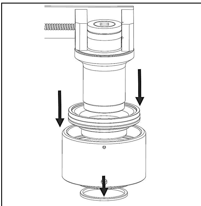
図 4.4 本体、ベアリングリング、インサートアセンブリの取り外し
