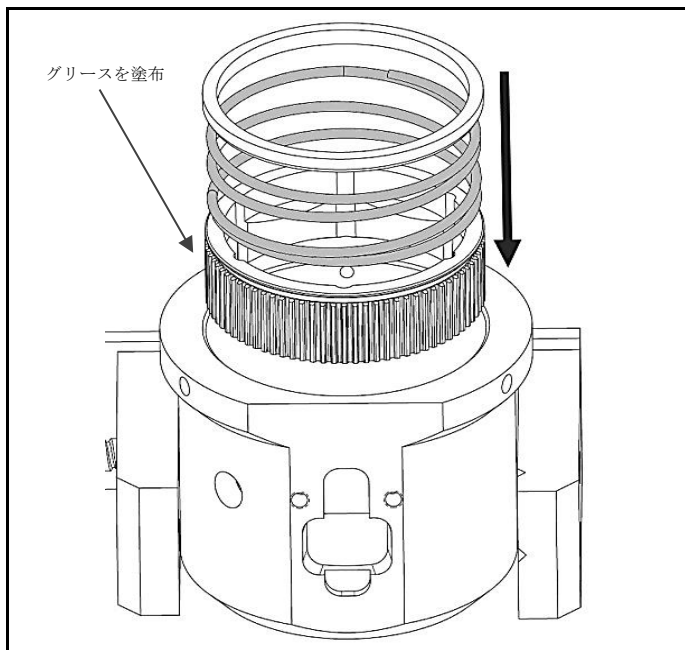
図 4.16 内部部品が正しく取り付けられていることの確認
