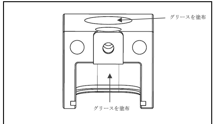
図 4.17 ギアボックスハウジングの準備
