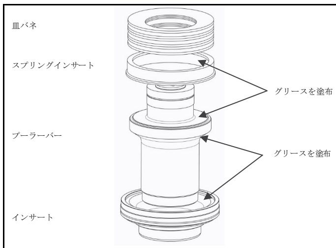
図 4.8 潤滑を追加する箇所
