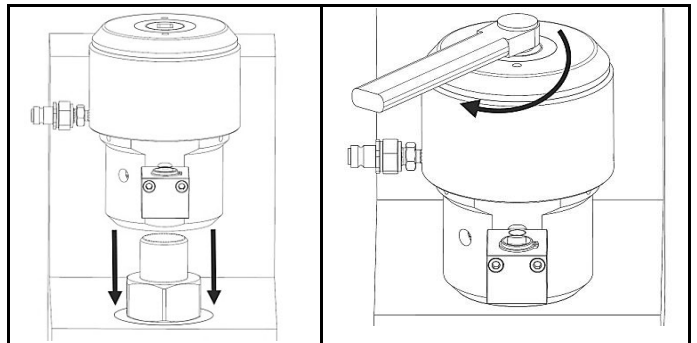
図 2.4 テンショナーの正しい位置決め
