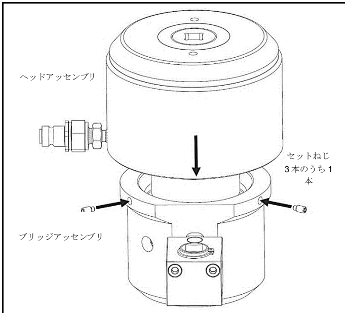
図 4.28 ヘッドアセンブリのブリッジアセンブリへの配置、グラブねじでの固定
