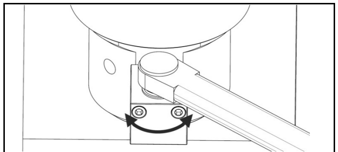
図 2.5 ギアボックスソケットの調整
