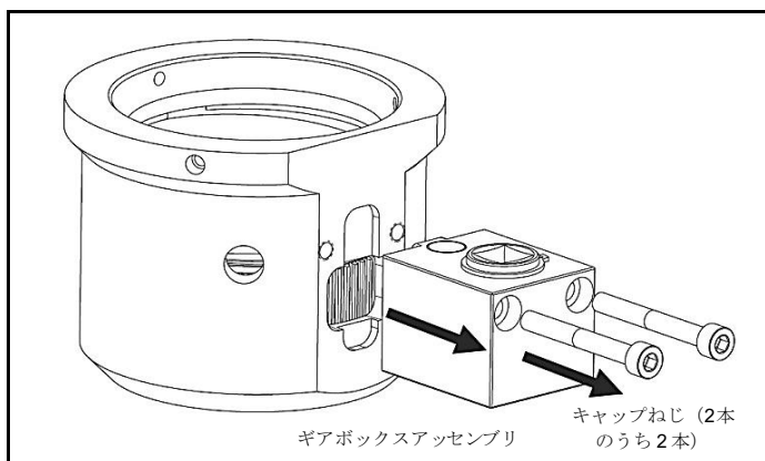
図 4.11 ブリッジアッセンブリとギアボックスアッセンブリの分離
