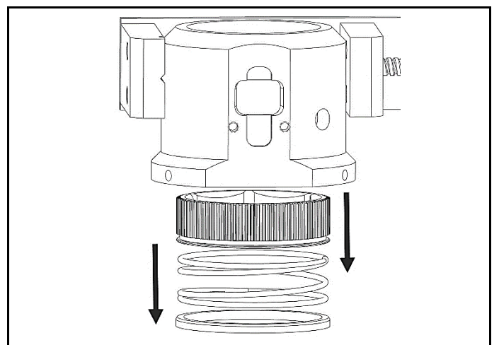
図 4.15 スプリングリテーナー、圧縮スプリング、ギア付きソケットの取り外し
