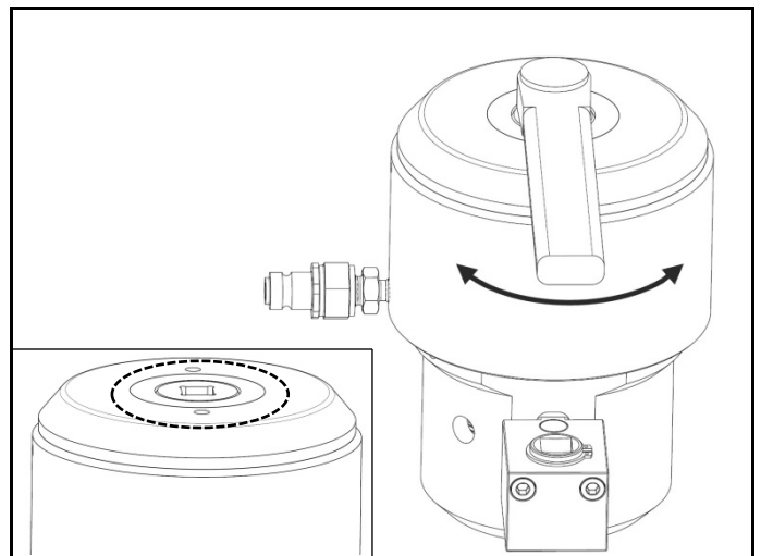
図 2.3 テンショナーの取り付け前確認
