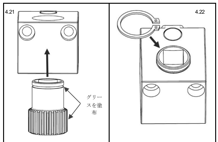
図 4.21 ドライブギアの準備および取り付け
