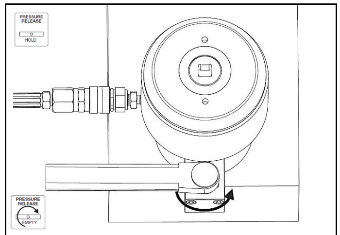
図 3.2 ギアボックスドライブを反時計回りに回す
