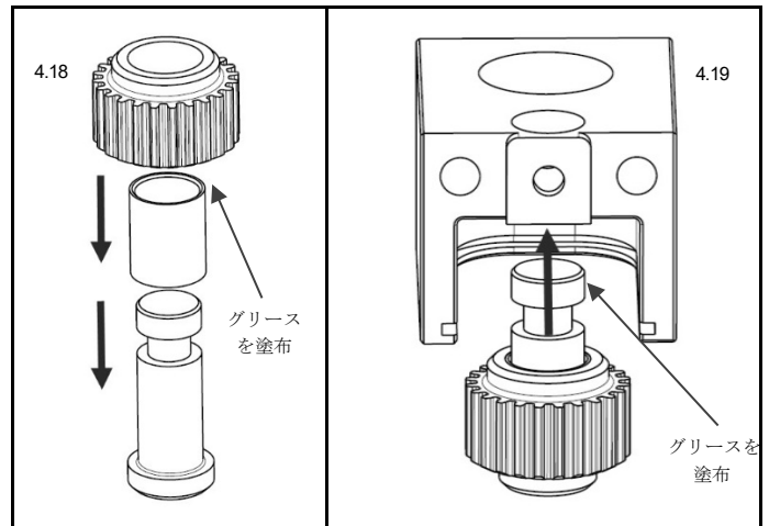
図 4.18 中間ギアの潤滑および組み立て
