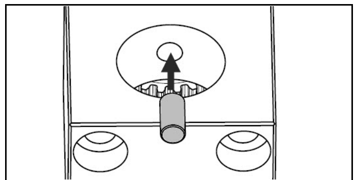
図 4.20 固定ダウエルピンの挿入
