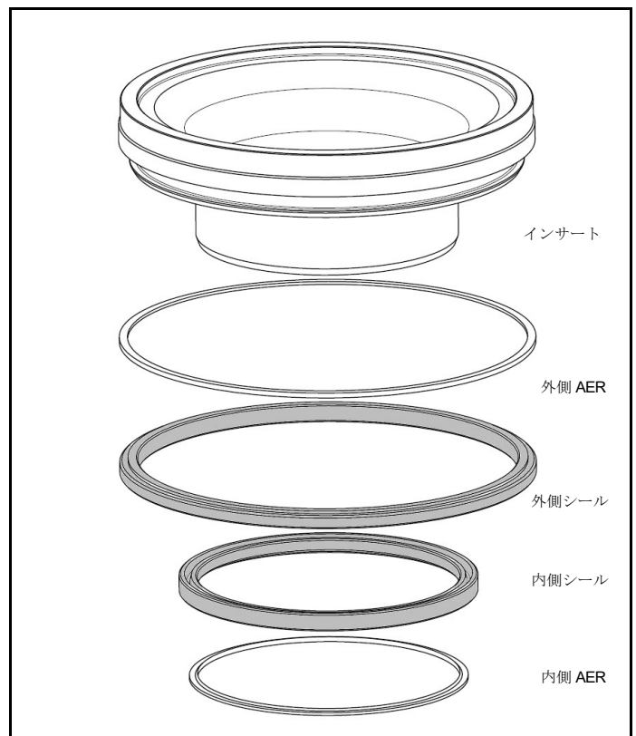
図 4.9 インサート、外側 AER／シール、内側 AER／シール
