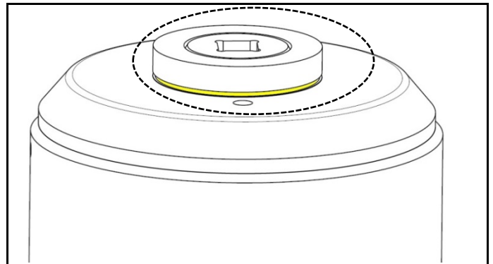
図 2.1 プーラーバーインジケーター溝
