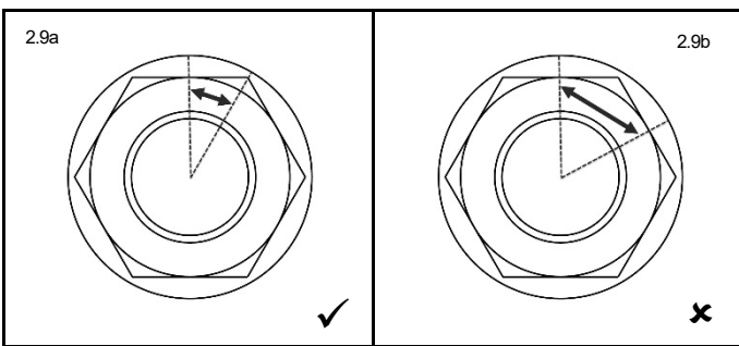
図 2.9a ボルトテンショニング完了
