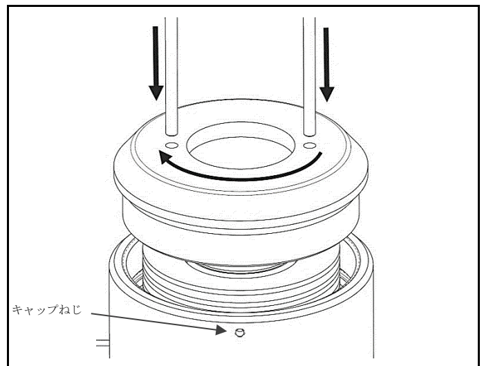
図 4.7 スプリングキャップの所定位置への固定
