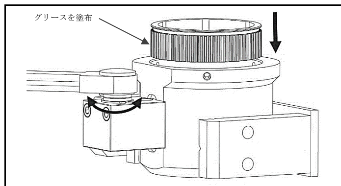
図 4.26 グリースの塗布、ギア付きソケットの挿入
