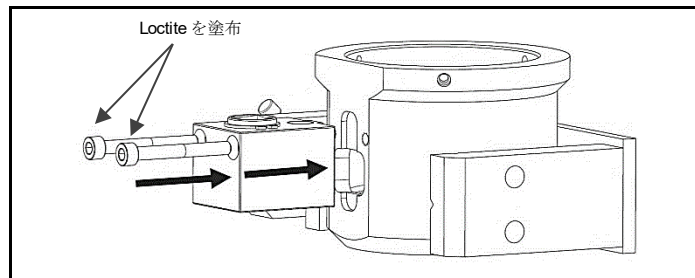
図 4.25 キャップねじへの Loctite の塗布、組み立てられたギアボックスのブリッジへの固定
