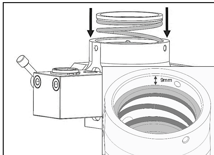
図 4.27 圧縮スプリングおよびスプリングリテーナーの挿入および固定
