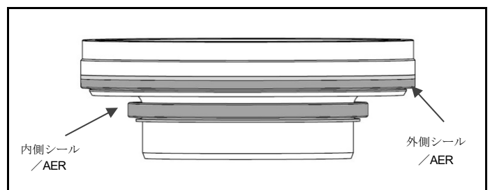
図 4.10 インサート、外側 AER／シール、内側 AER／シール（組み立て状態）
