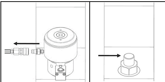
図 2.8 ホースの取り外し、テンショナーを次のボルトへ移動
