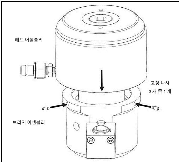
그림 4.28 헤드 어셈블리를 브리지 어셈블리에 배치, 그라브 나사로
