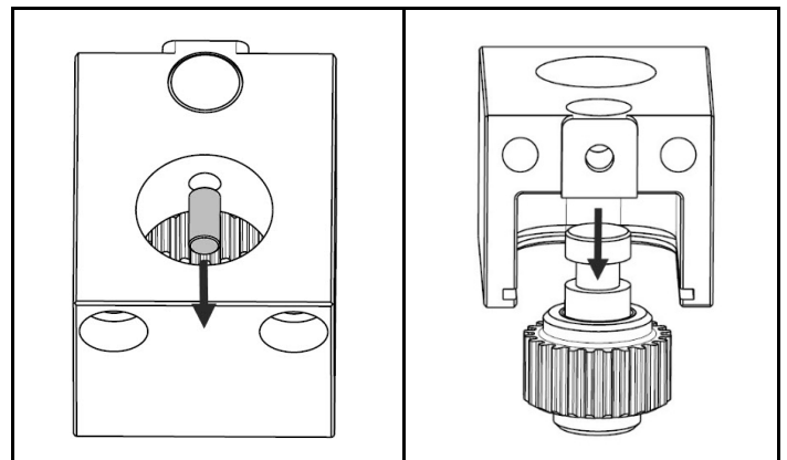
그림 4.14 고정 다웰 핀을 제거한 후 중간 기어 어셈블리 제거
