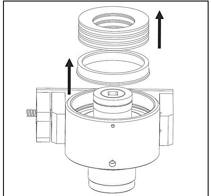
그림 4.3 디스크 스프링과 스프링 인서트 제거
