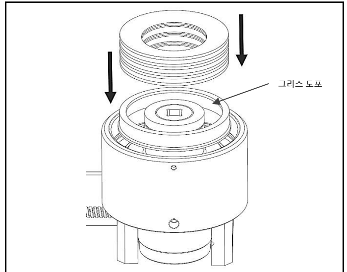
그림 4.6 스프링 인서트 및 디스크 스프링 삽입. 주의하여 올바르게 쌓기
