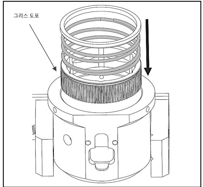
그림 4.16 내부 부품이 올바르게 맞춰졌는지 점검
