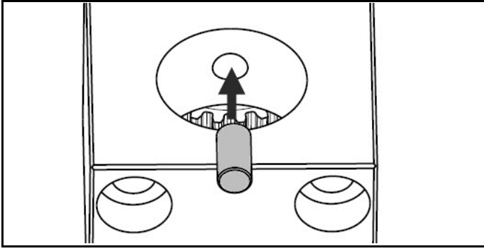
그림 4.20 고정 다웰 핀 삽입
