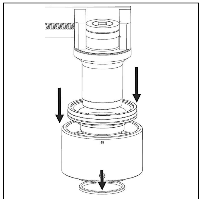
그림 4.4 본체, 베어링 링, 인서트 어셈블리 제거
