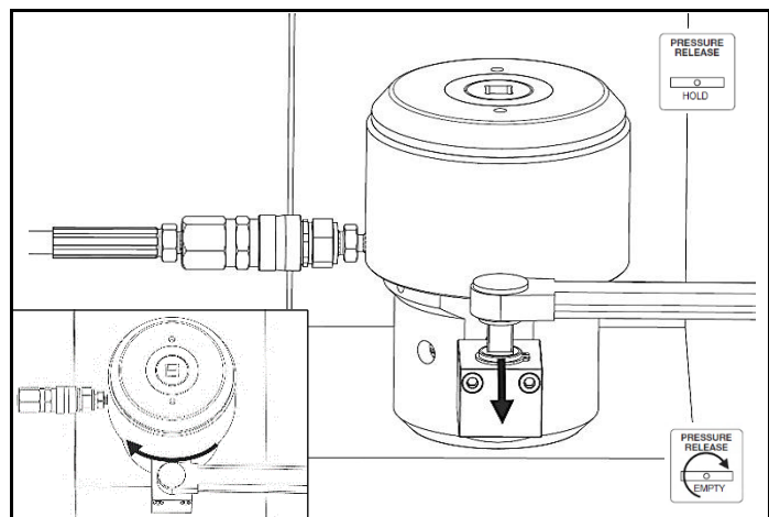
그림 2.7 기어박스 드라이브를 돌려 너트 조이기
