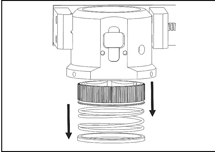
그림 4.15 스프링 리테이너, 압축 스프링 및 기어드 소켓 제거
