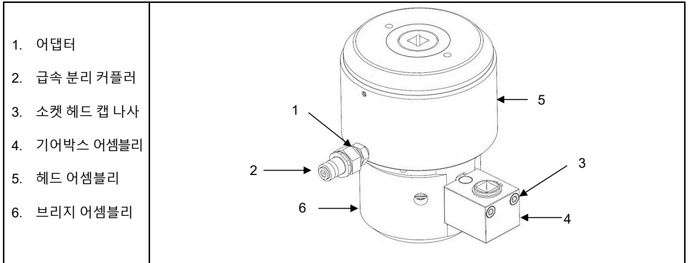
그림 1.1 PGT 시리즈 싱글 스테이지 텐서너의 주요 기능 및 구성품
