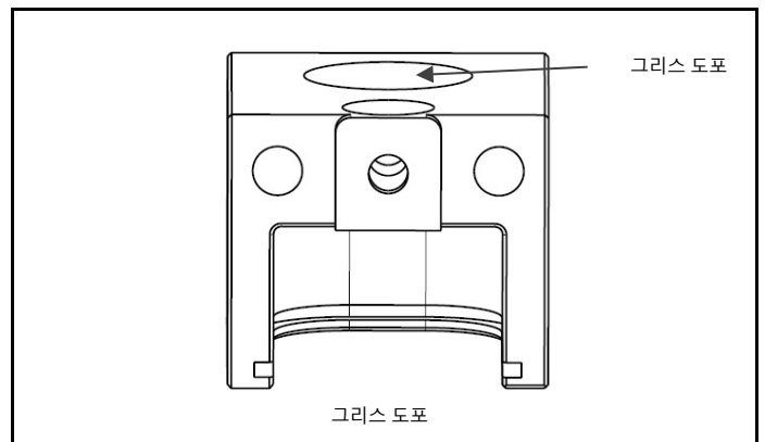
그림 4.17 기어박스 하우징 준비
