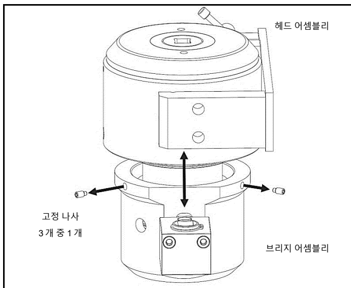
그림 4.1 헤드 어셈블리 및 브리지 어셈블리의 분리
