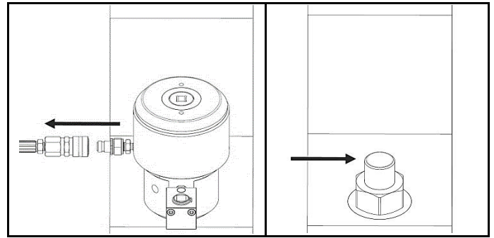
그림 2.8 호스 분리, 텐서너를 다음 볼트로 이동
