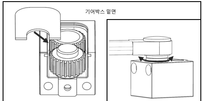
그림 4.24 기어박스 커버 장착, 기어가 원활하게 움직이는지 점검
