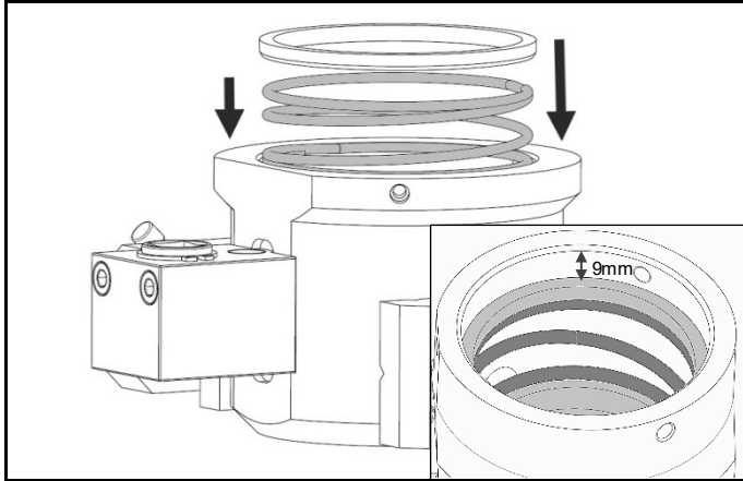
그림 4.27 압축 스프링 및 스프링 리테이너 삽입 및 고정
