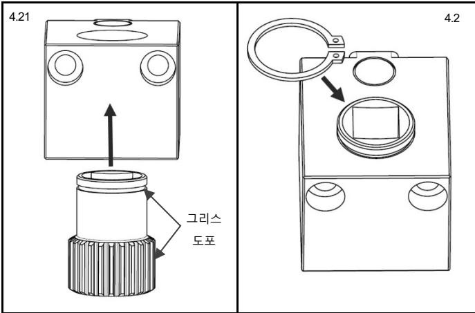
그림 4.21 드라이브 기어 준비 및 설치
