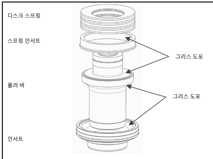
그림 4.8 추가 윤활 영역
