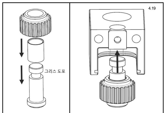
그림 4.18 중간 기어 윤활 및 조립
