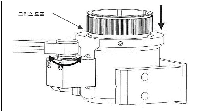
그림 4.26 그리스 도포, 기어드 소켓 삽입
