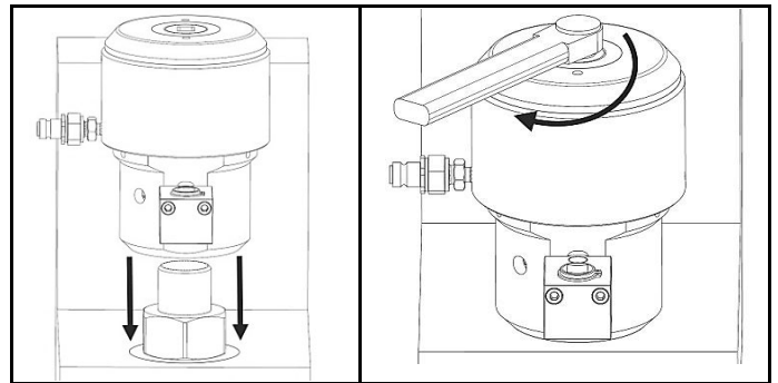
그림 2.4 텐서너의 올바른 위치
