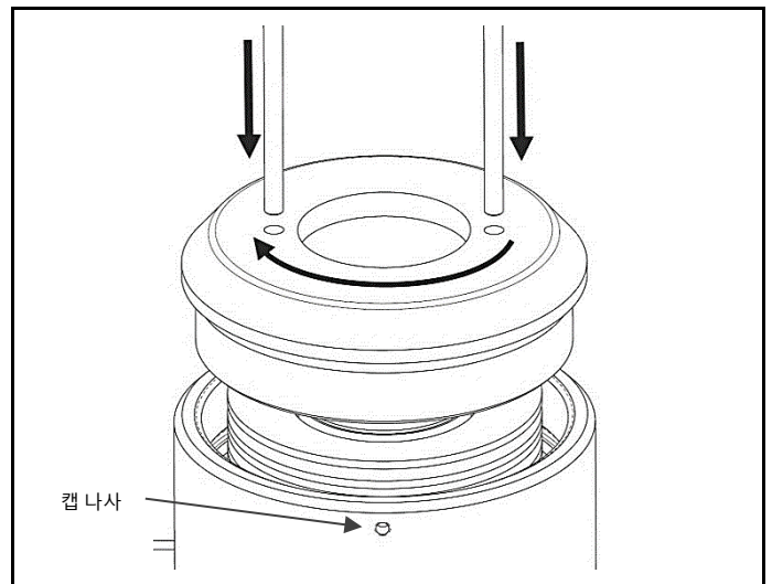
그림 4.7 스프링 캡을 제자리에 고정하기
