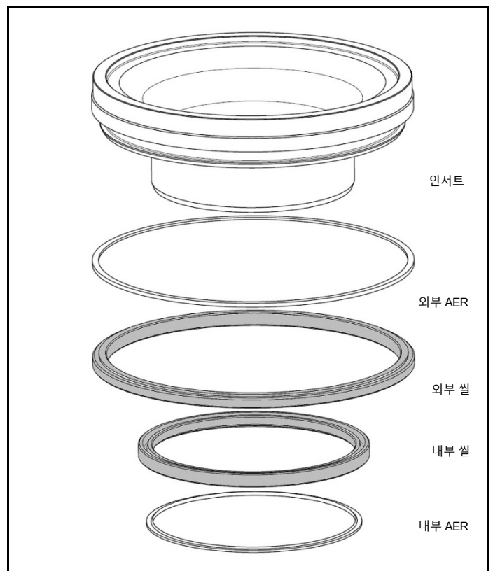
그림 4.9 인서트, 외부 AER/실, 내부 AER/실
