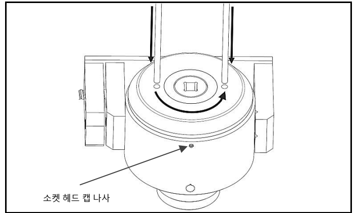
그림 4.2 토미 바를 사용하여 스프링 캡 제거
