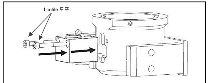
그림 4.25 캡 나사에 Loctite 도포, 조립된 기어박스를 브리지에 고정
