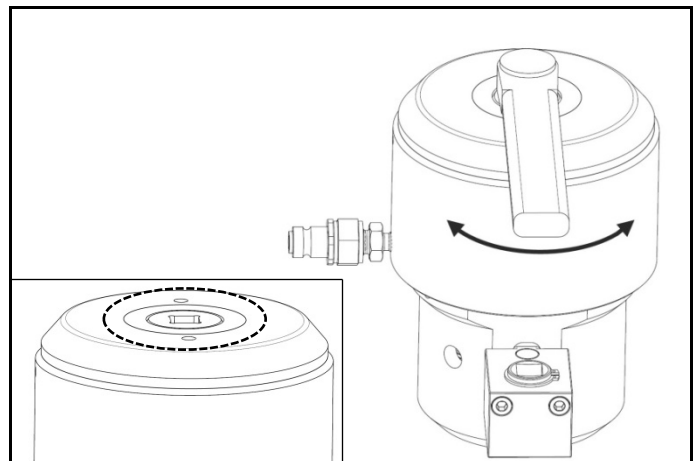
그림 2.3 설치 전 텐서너 점검
