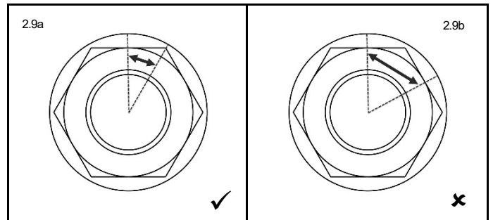
그림 2.9a 볼트 텐서닝 완성
