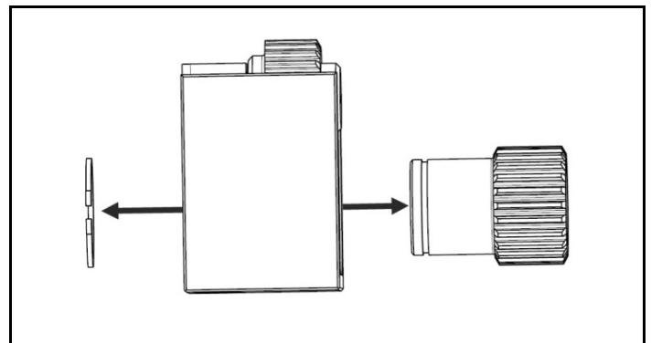
그림 4.13 드라이브 기어 서클립과 드라이브 기어 제거
