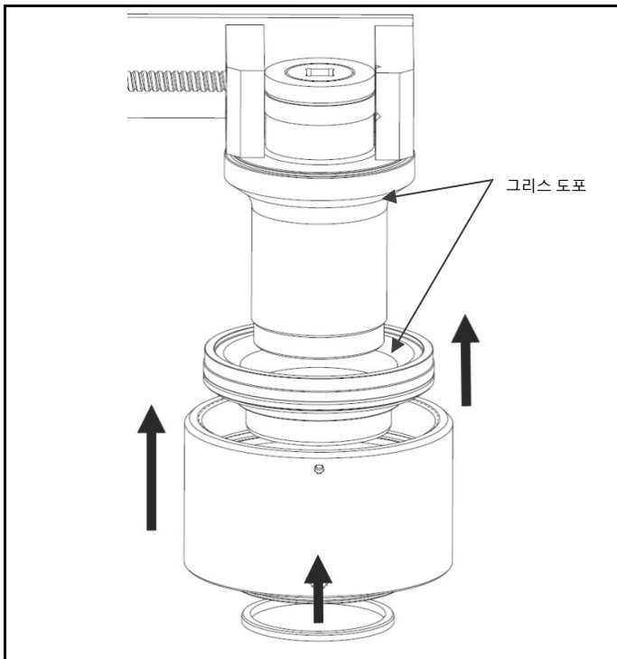
그림 4.5 인서트 어셈블리, 본체 및 베어링 링을 풀러 바에 장착하기
