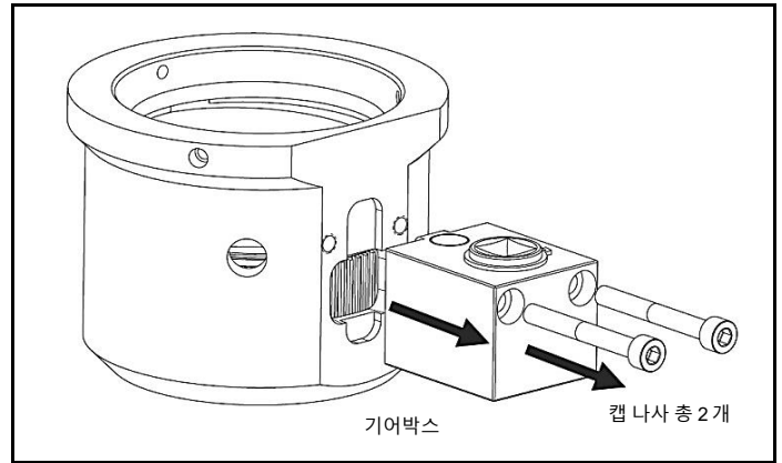
그림 4.11 브리지 어셈블리 및 기어박스 어셈블리의 분리
