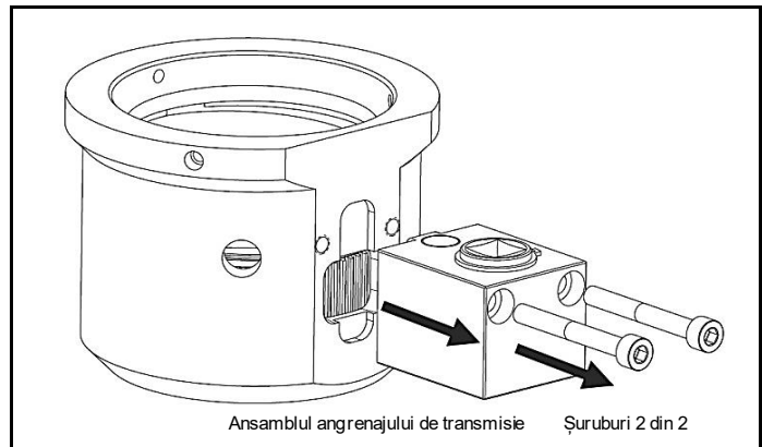
Fig. 4.11 Separarea ansamblului punții și ansamblului angrenajului de transmisie
