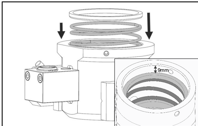
Fig. 4.27 Introduceți și fixați arcul de compresie și elementul de reținere a arcului (dacă este folosit)
