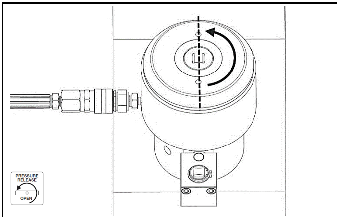
Fig. 3.1 Strângeți bara extractoare înapoi 3/4 de tură
