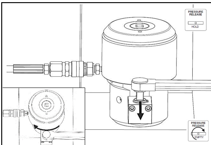
Fig. 2.7 Rotiți angrenajul de transmisie pentru a strânge piulița
