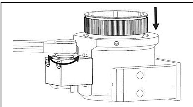
Fig. 4.26 Aplicați vaselină, introduceți racordul angrenat
