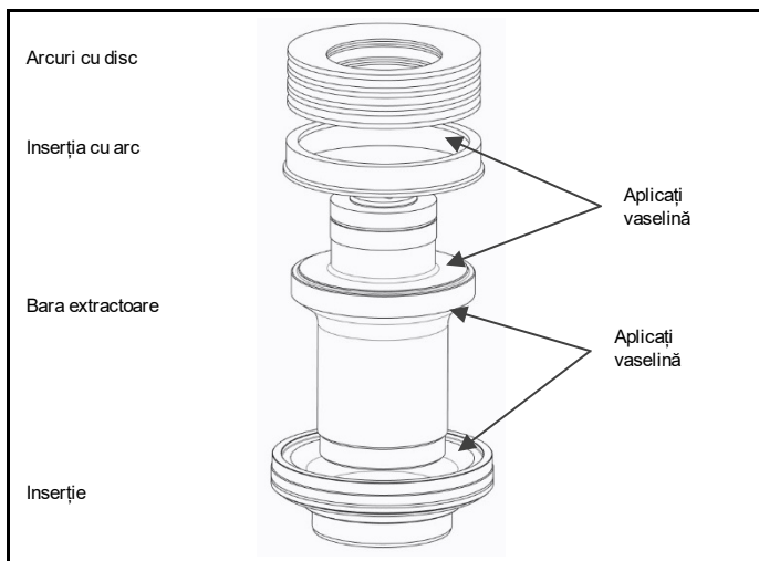
Fig. 4.8 Zonele care pot necesita lubrifiere suplimentară
