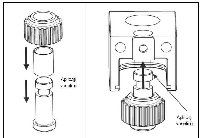
Fig. 4.18 Gresați și asamblați angrenajul intermediar
