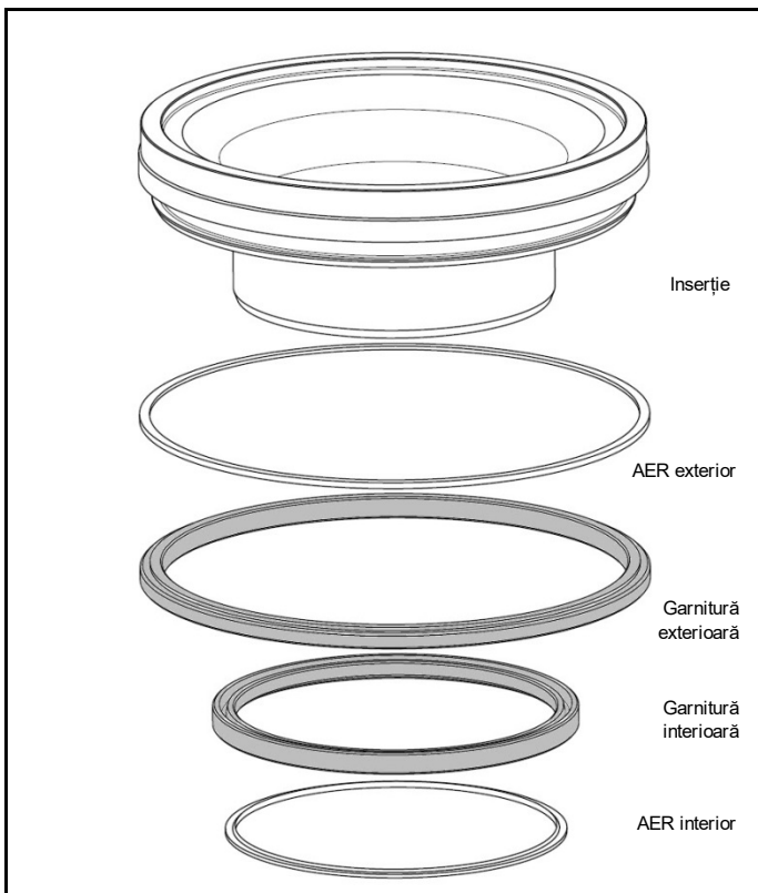
Fig. 4.9 Inserție, AER/ garnitură exterior(-oară), AER/ garnitură interior(-oară)
