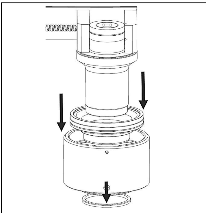
Fig. 4.4 Demontați corpul, inelul, ansamblul
