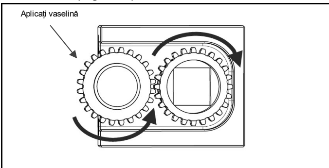
Fig. 4.23 Verificați ca angrenajele montate să funcționeze lin și aplicați vaselină
