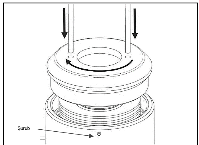
Fig. 4.7 Fixați capul cu arc la locul său
