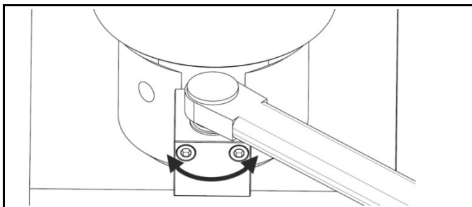
Fig. 2.5 Reglați racordul angrenajului de transmisie
