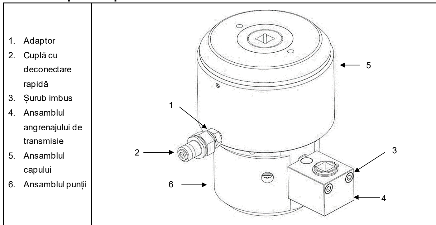
Fig. 1.1 Caracteristicile și componentele principale ale dispozitivelor de tensionare din seria PGT cu punte simplă
