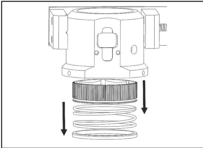
Fig. 4.15 Demontați elementul de reținere a arcului (dacă este folosit), arcurile de compresie și racordul angrenajului de transmisie
