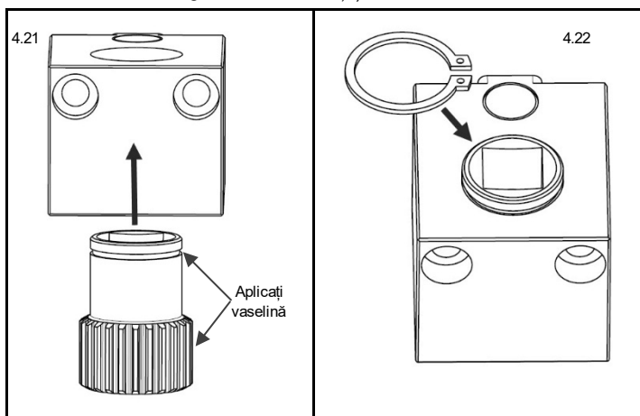
Fig. 4.21 Pregătiți și instalați angrenajul de transmisie
