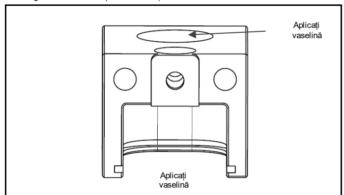
Fig. 4.17 Pregătiți carcasa angrenajului de transmisie
