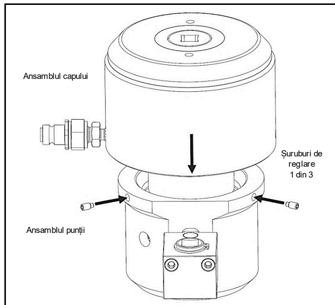
Fig. 4.28 Fixați ansamblul capului pe ansamblul punții, fixați cu șuruburi autofiletante
