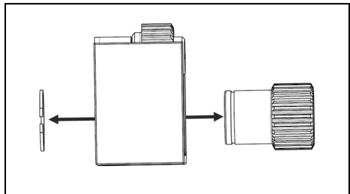
Fig. 4.13 Demontați inelul elastic al angrenajului de transmisie și angrenajul de transmisie
