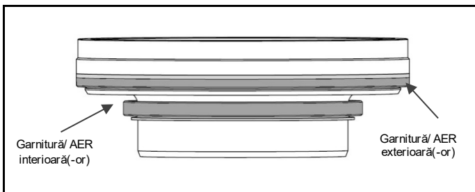
Fig. 4.10 Inserție, AER/ garnitură exterior(-oară), AER/ garnitură interior(-oară) asamblată
