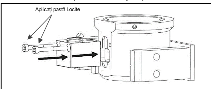
Fig. 4.25 Aplicați pastă Loctite pe șuruburi, fixați angrenajul de transmisie asamblat pe punte
