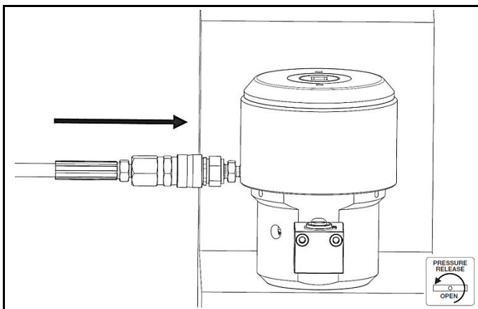
Fig. 2.6 Conectarea furtunului
