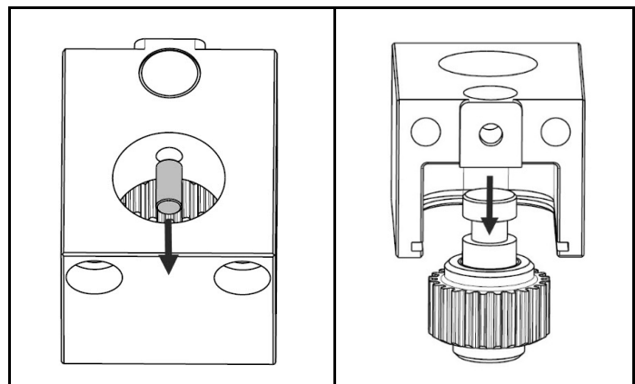
Fig. 4.14 Demontați știftul de fixare, apoi ansamblul angrenajului intermediar
