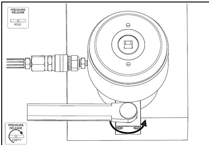
Fig. 3.2 Rotiți angrenajul de transmisie în sens antiorar
