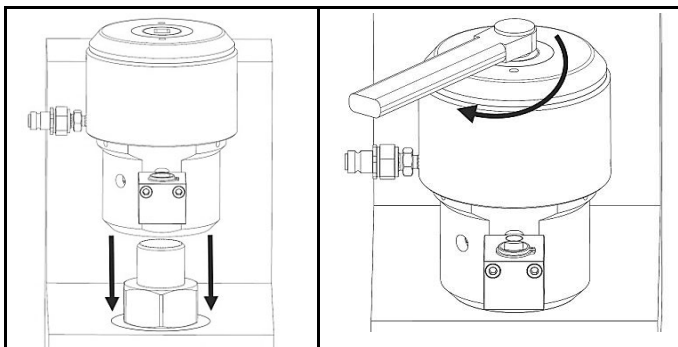
Fig. 2.4 Poziționarea corectă a dispozitivului de tensionare
