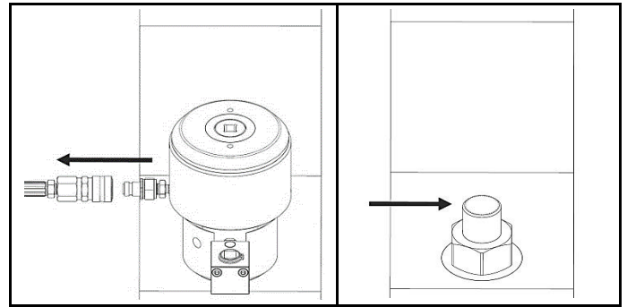
Fig. 2.8 Scoateți furtunul, mutați dispozitivul de tensionare pe următorul bolt
