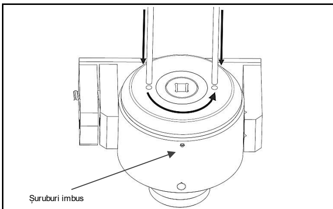
Fig. 4.2 Scoateți capacul cu arc cu ajutorul levierelor
