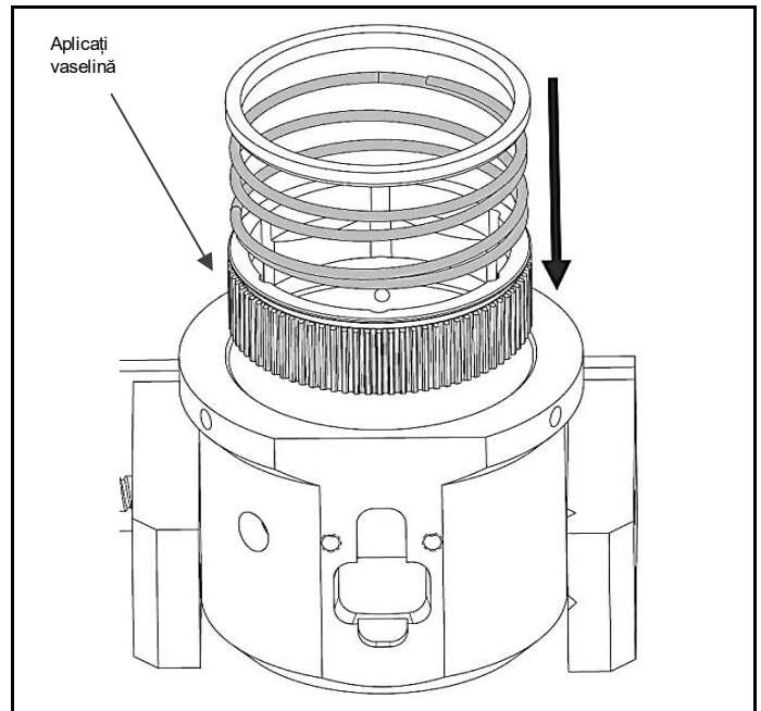
Fig. 4.16 Verificați dacă componentele interne sunt fixate corect
