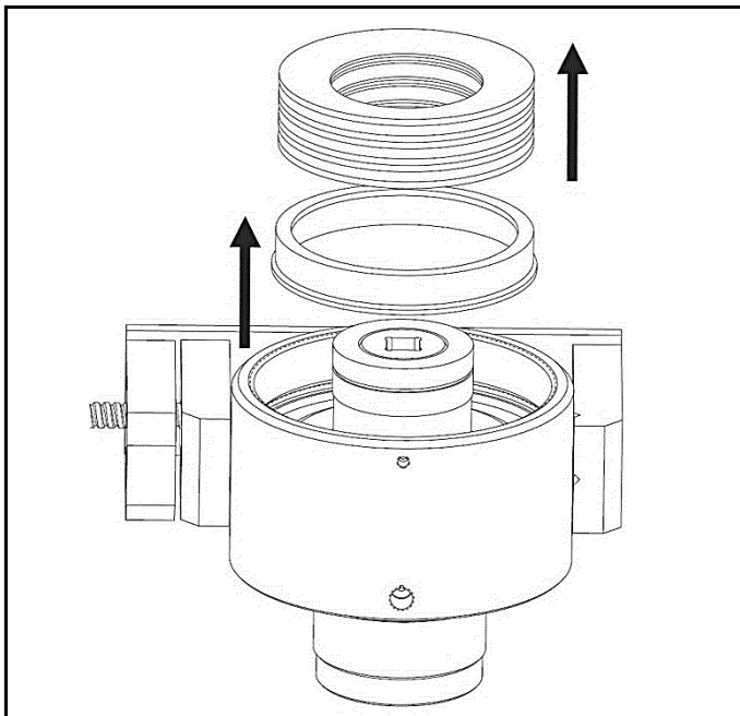
Fig. 4.3 Demontați arcurile cu disc și inserția cu disc
