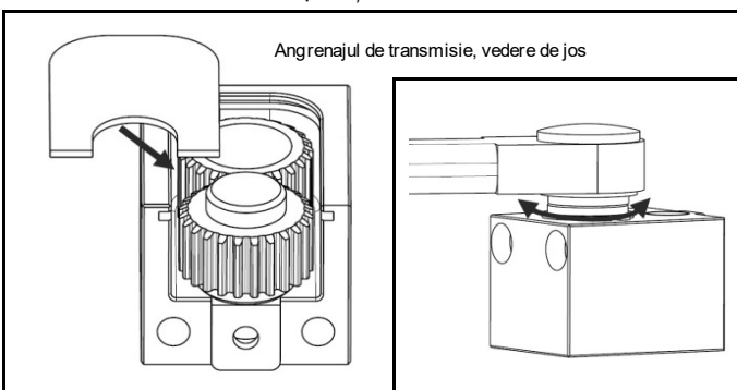
Fig. 4.24 Fixați capacul angrenajului de transmisie, verificați funcționarea lină a angrenajelor
