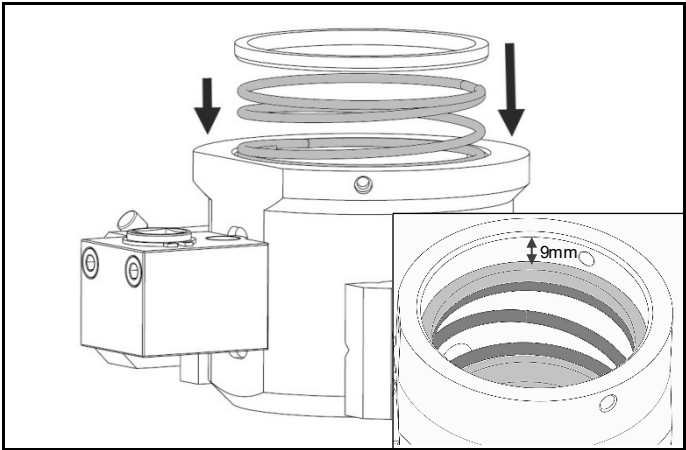
图 4.27 插入并固定压缩弹簧和弹簧固定器
