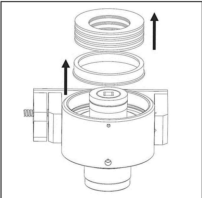
图 4.3 拆下盘式弹簧和弹簧插件
