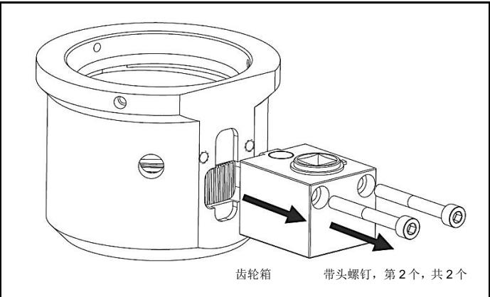
图 4.11 座桥总成和齿轮箱总成分离
