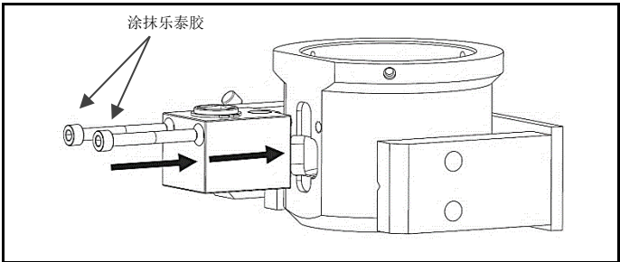
图 4.25 螺钉涂抹乐泰胶，将组装的齿轮箱固定到座桥上
