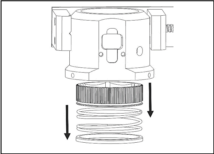
图 4.15 拆下弹簧固定器、压簧和带齿套筒头
