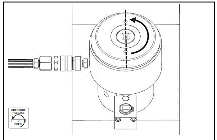
图 3.1 将拉杆回旋 3/4 圈
