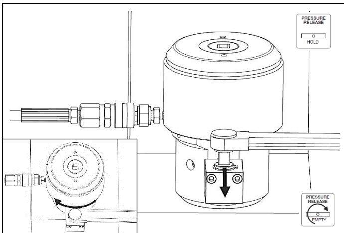
图 2.7 转动齿轮箱传动以拧紧螺母
