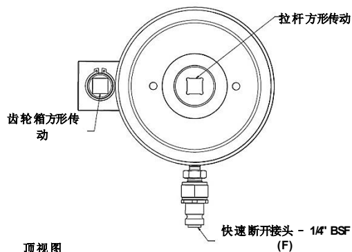
顶视图
