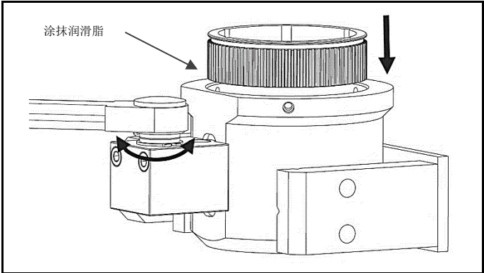
图 4.26 涂抹润滑脂，插入带齿套筒头
