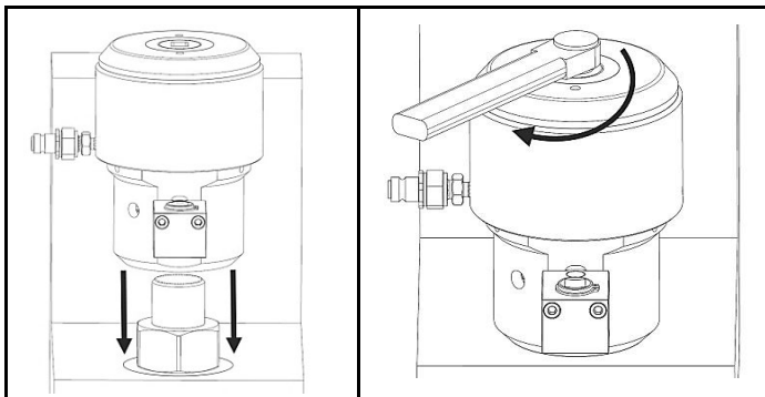
图 2.4 拉伸器正确就位
