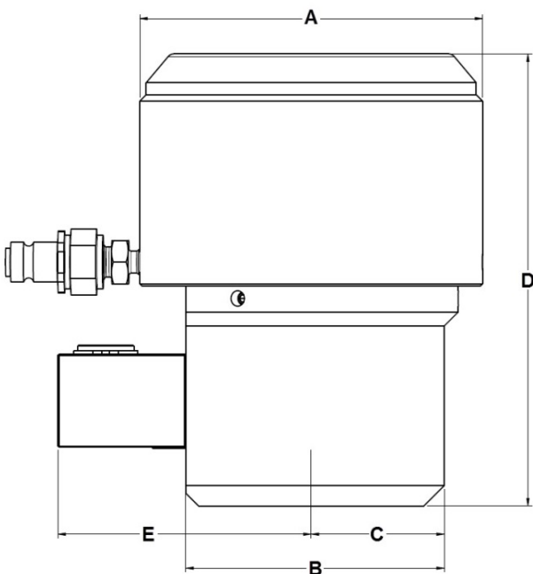
侧视图
