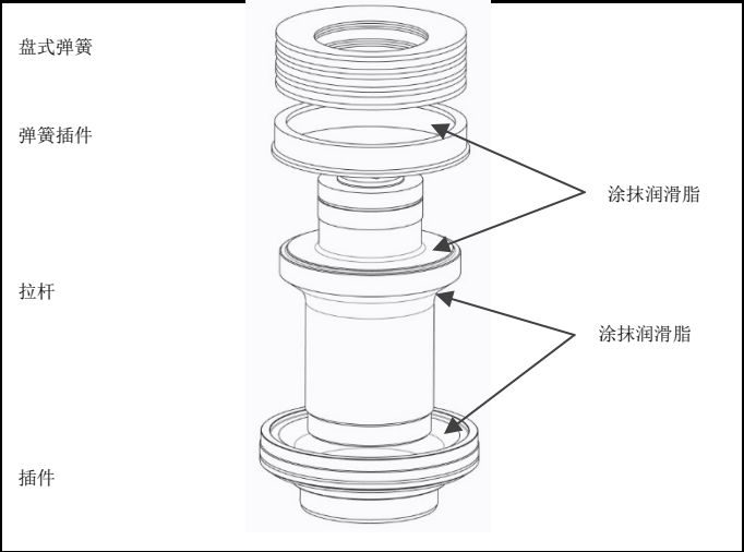
图 4.8 额外润滑的区域
