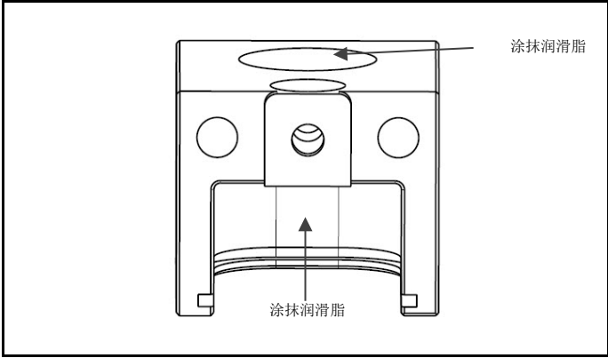
图 4.17 准备齿轮箱外壳
