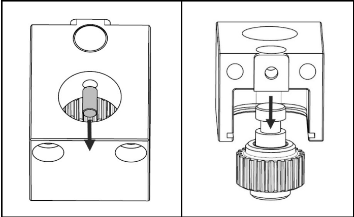
图 4.14 拆下定位销，然后拆下中间齿轮
