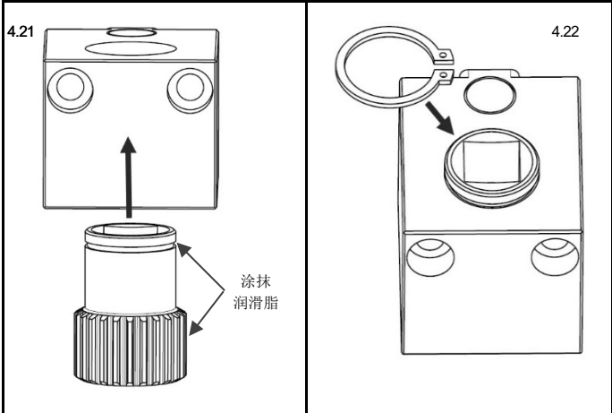
图 4.21 准备并安装传动齿轮
