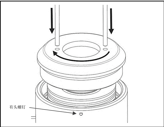
图 4.7 将弹簧帽固定到位
