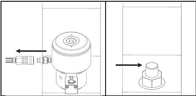
图 2.8 断开软管，将拉伸器转移至下一螺栓
