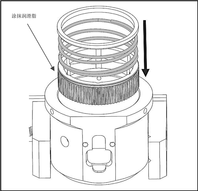
图 4.16 检查内部部件是否正确装配
