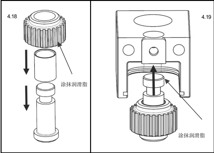
图 4.18 涂抹润滑脂并组装中间齿轮
