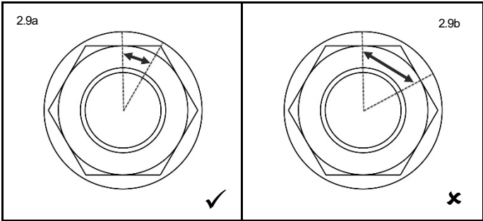
图 2.9a 螺栓旋紧已完成
