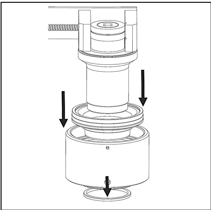
图 4.4 拆下拉伸头本体、轴承环和插件总成
