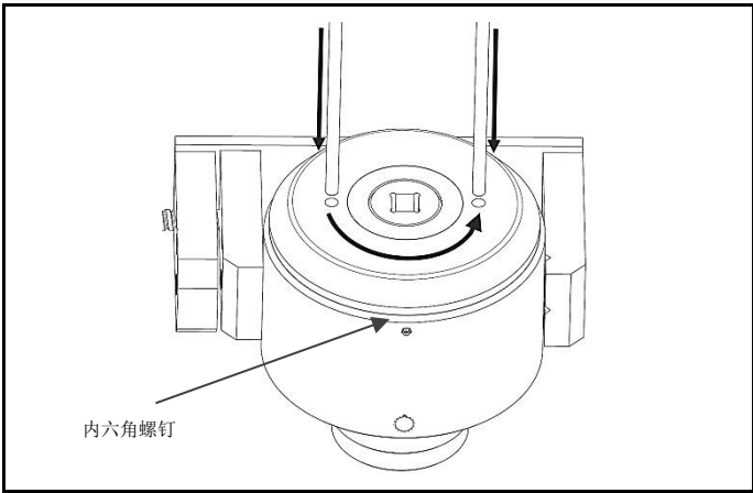
图 4.2 使用旋杆拆下弹簧帽
