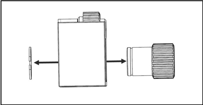
图 4.13 拆下传动齿轮卡环和传动齿轮
