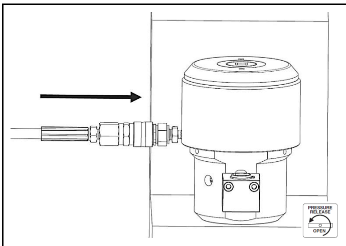
图 2.6 软管接头
