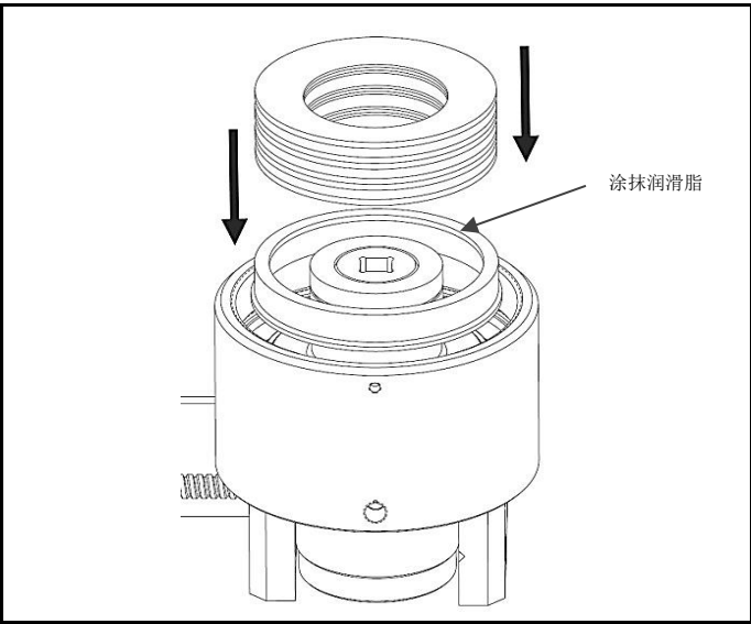
图 4.6 插入弹簧插件和盘式弹簧，注意弹簧正确堆叠
