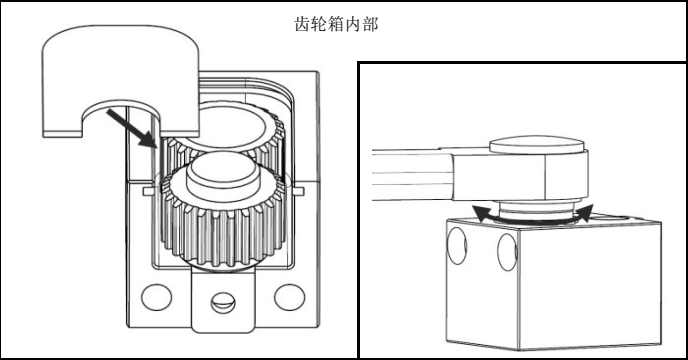
图 4.24 安装齿轮箱盖板，检查齿轮是否可以无阻碍转动
