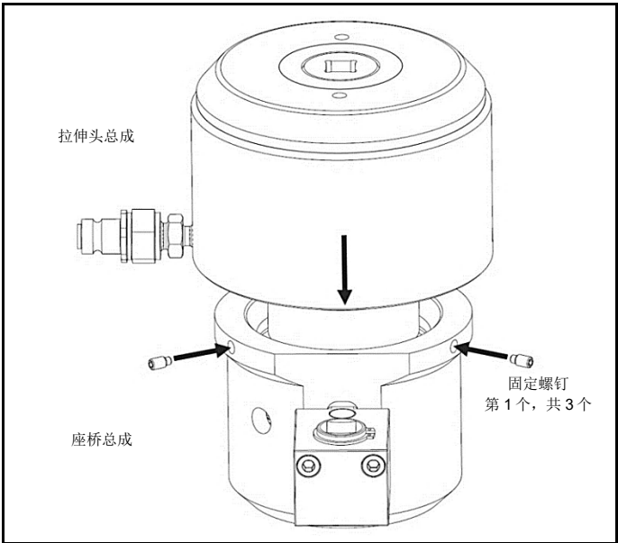
图 4.28 将拉伸头总成放置到座桥总成上，使用平头螺钉固定
