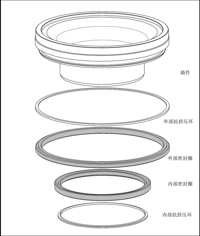
图 4.9 插件、外部抗挤压环/密封圈、内部抗挤压环/密封圈
