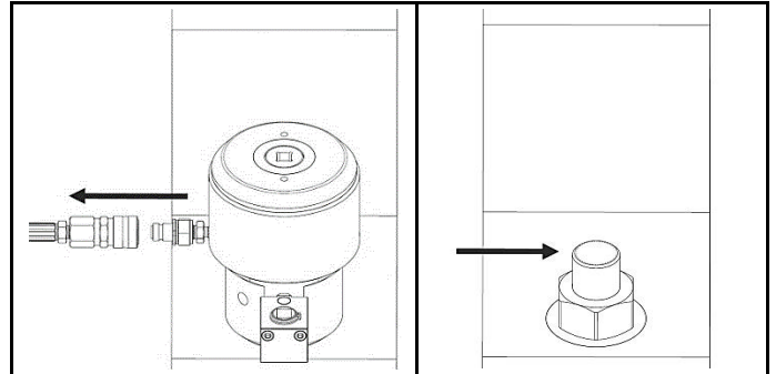
Fig. 2.8 Débrancher le flexible, déplacer le tendeur sur le boulon suivant
