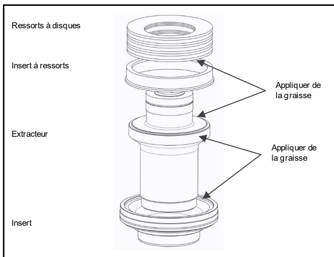
Fig. 4.8 Zones de lubrification complémentaire
