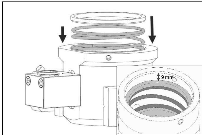
Fig. 4.27 Introduire et fixer le ressort de compression et l'attache du ressort (si utilisée)
