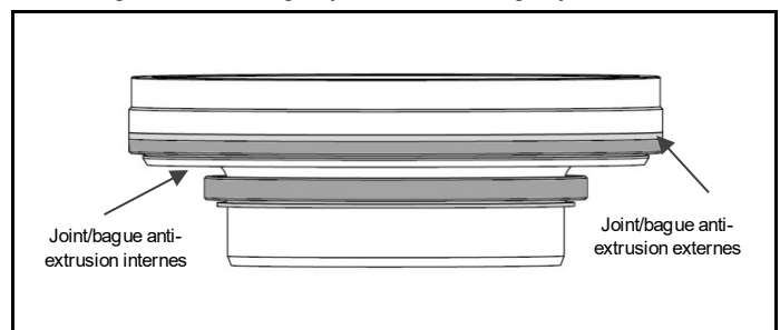
Fig. 4.10 Insert, bague/joint externes et bague/joint internes assemblés
