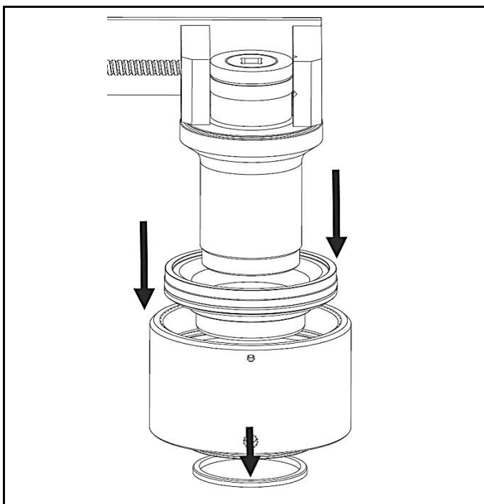
Fig. 4.4 Retirer le corps, la bague de roulement, l'insert
