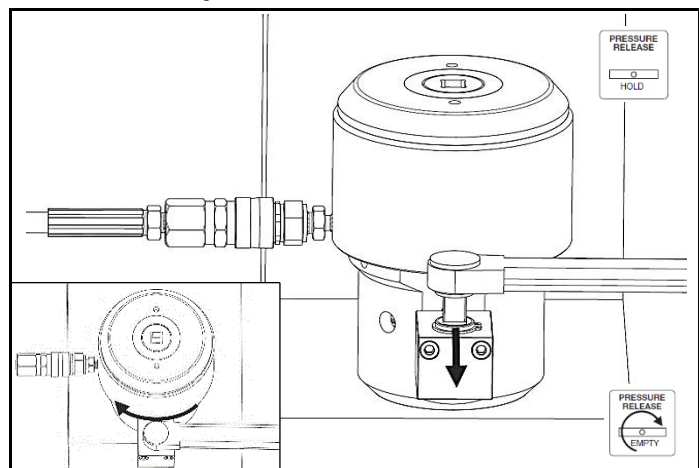
Fig. 2.7 Tourner l'entraînement de la boîte d'engrenages pour serrer l'écrou
