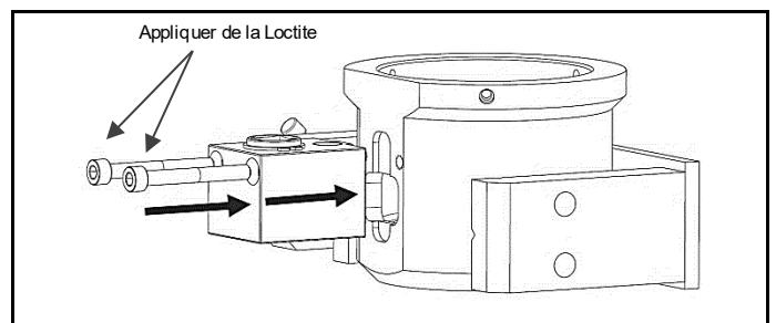
Fig. 4.25 Appliquer de la Loctite sur les vis creuses ; fixer la boîte d'engrenages assemblée sur le pont
