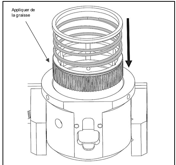
Fig. 4.16 Vérifier que les pièces internes correspondent bien
