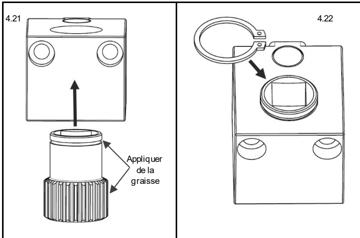
Fig. 4.21 Préparer et installer le pignon d'entraînement
