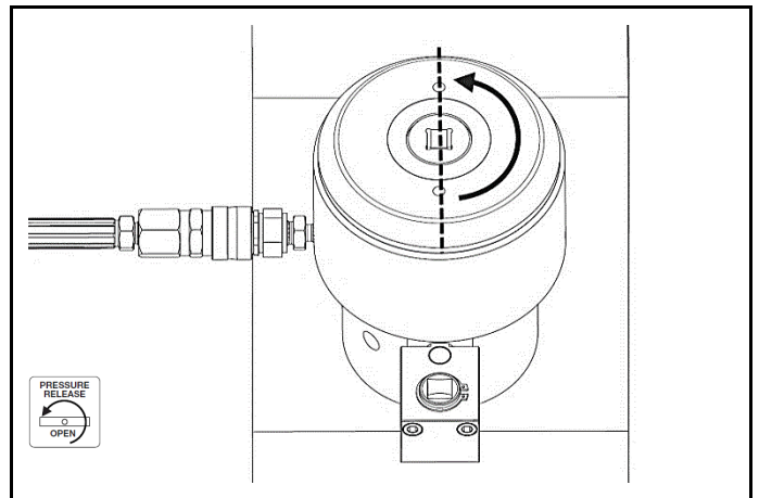
Fig. 3.1 Tourner l'extracteur de 3/4 de tour en sens inverse
