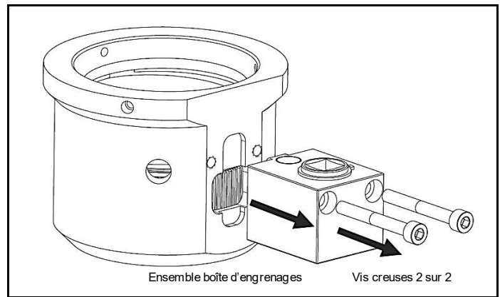
Fig. 4.11 Séparation des ensembles pont et boîte d'engrenages
