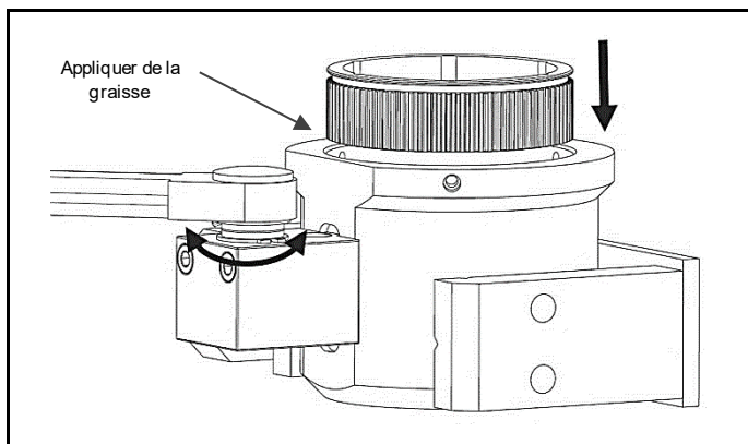
Fig. 4.26 Appliquer de la graisse ; introduire la douille à engrenage
