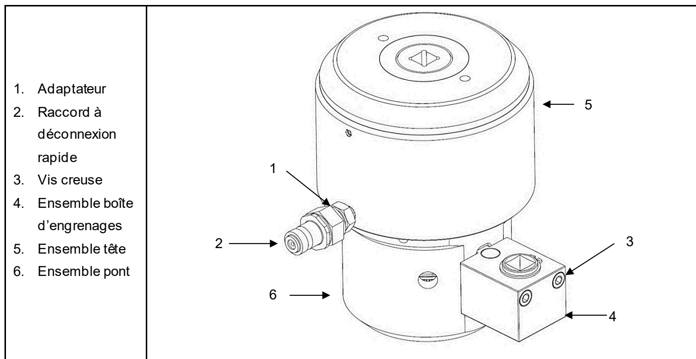
Fig. 1.1 Caractéristiques et composants principaux des tendeurs à étage simple de la série PGT
