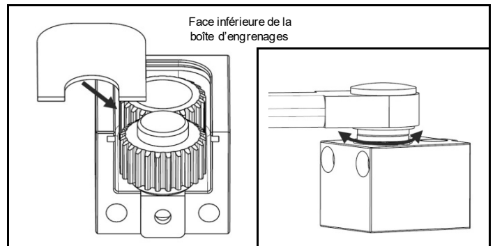
Fig. 4.24 Installer le couvercle de la boîte d'engrenages ; vérifier que les pignons tournent correctement
