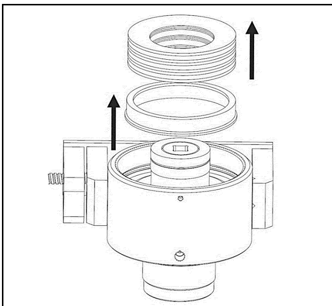
Fig. 4.3 Retirer les ressorts à disques et l'insert à ressorts
