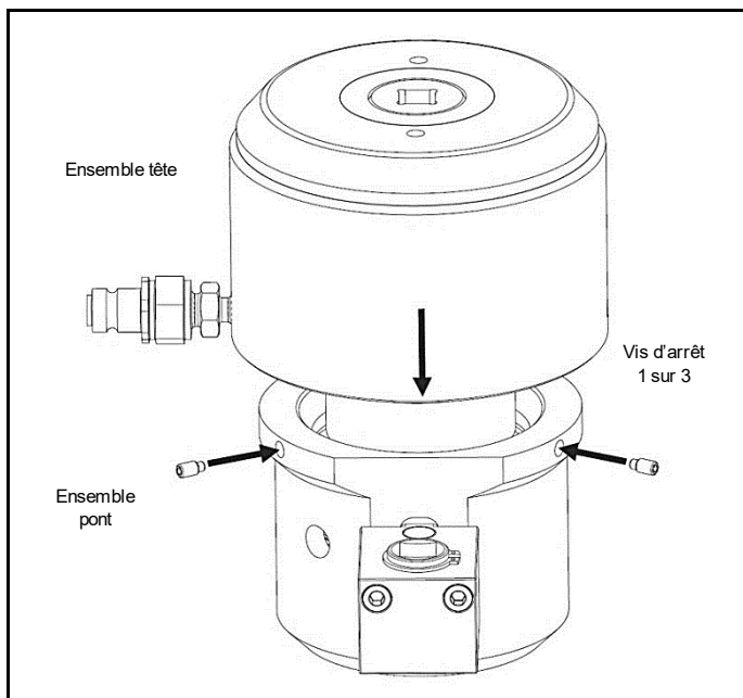
Fig. 4.28 Placer l'ensemble tête sur l'ensemble pont ; fixer avec des vis sans tête
