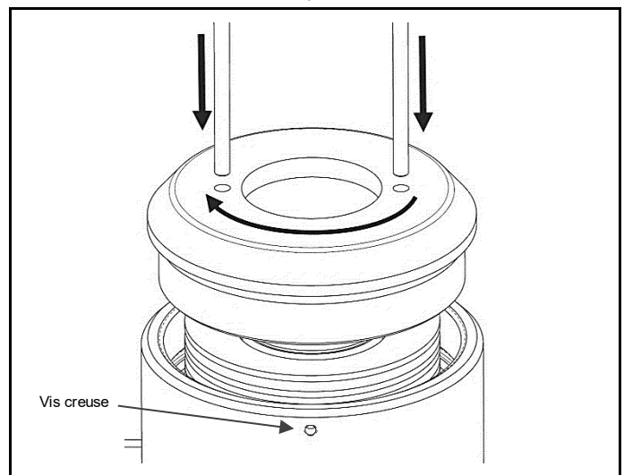
Fig. 4.7 Fixer le bouchon à ressort
