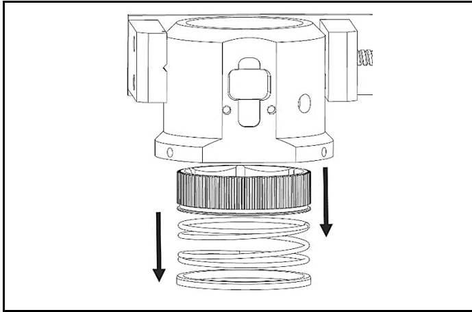
Fig. 4.15 Retirer l'attache du ressort (si utilisée), les ressorts de compression et la douille à engrenage
