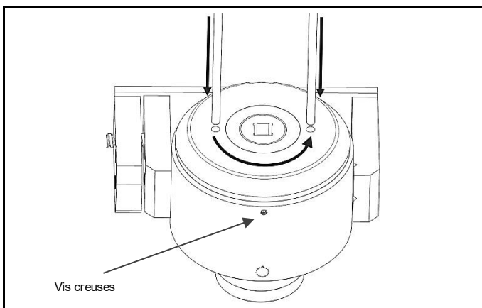
Fig. 4.2 Utiliser des broches de manœuvre pour retirer le bouchon à ressort
