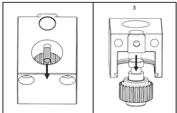
Fig. 4.14 Retirer la goupille d'immobilisation, suivie de l'ensemble du pignon intermédiaire
