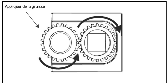
Fig. 4.23 Vérifier que les pignons assemblés tournent correctement ; appliquer de la graisse
