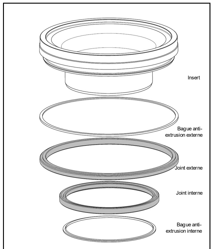
Fig. 4.9 Insert, bague/joint externes, bague/joint internes
