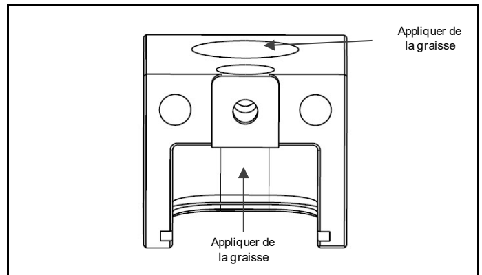
Fig. 4.17 Préparer le logement de la boîte d'engrenages
