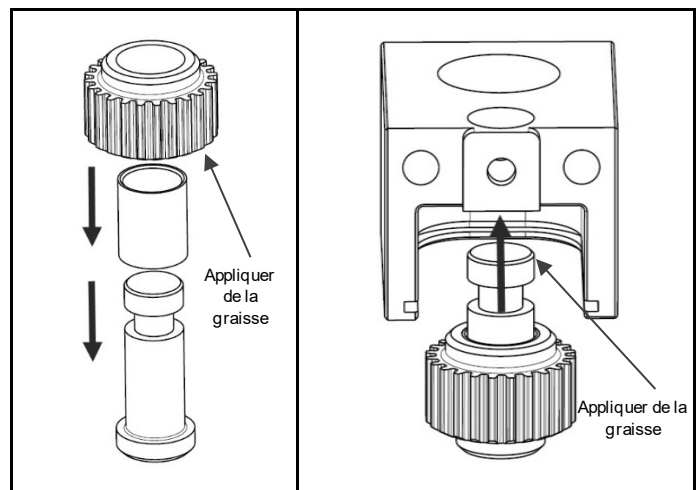
Fig. 4.18 Graisser et assembler le pignon intermédiaire
