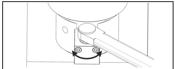
Fig. 2.5 Ajuster la douille de la boîte d'engrenages
