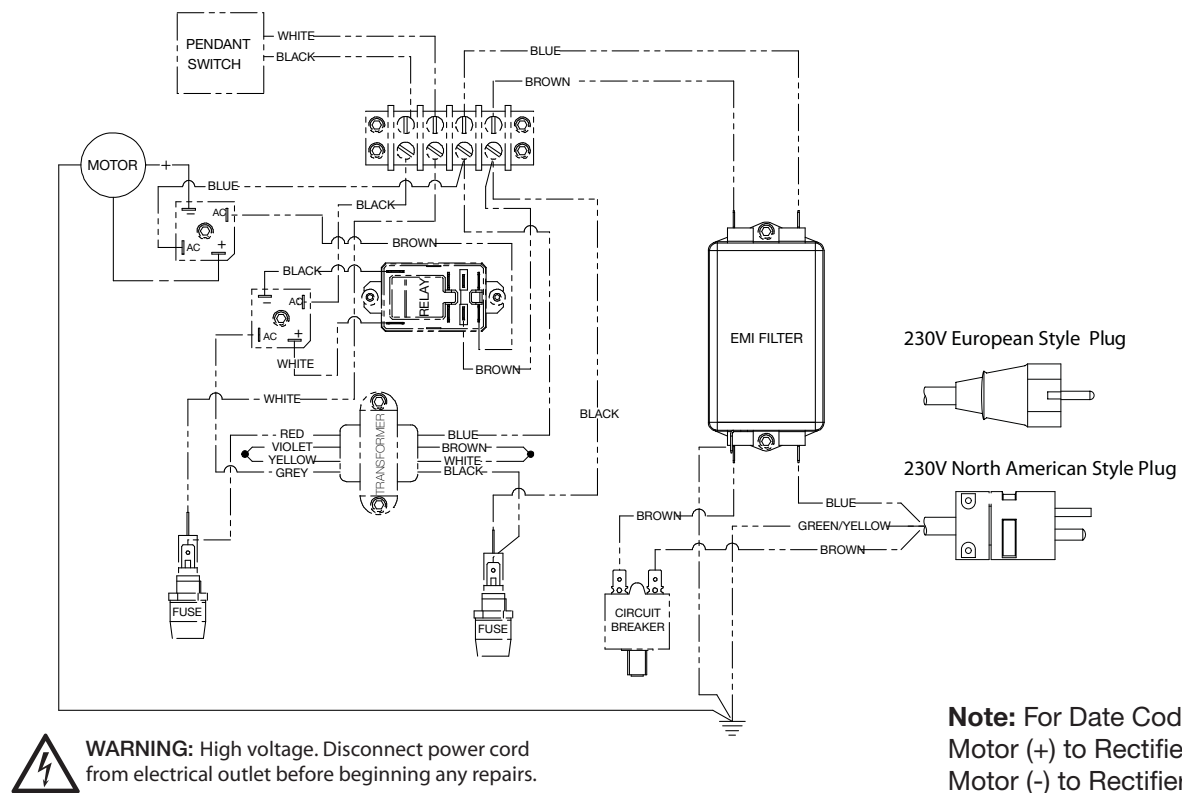
Figure 20 - 230 Volt Wiring Diagram
