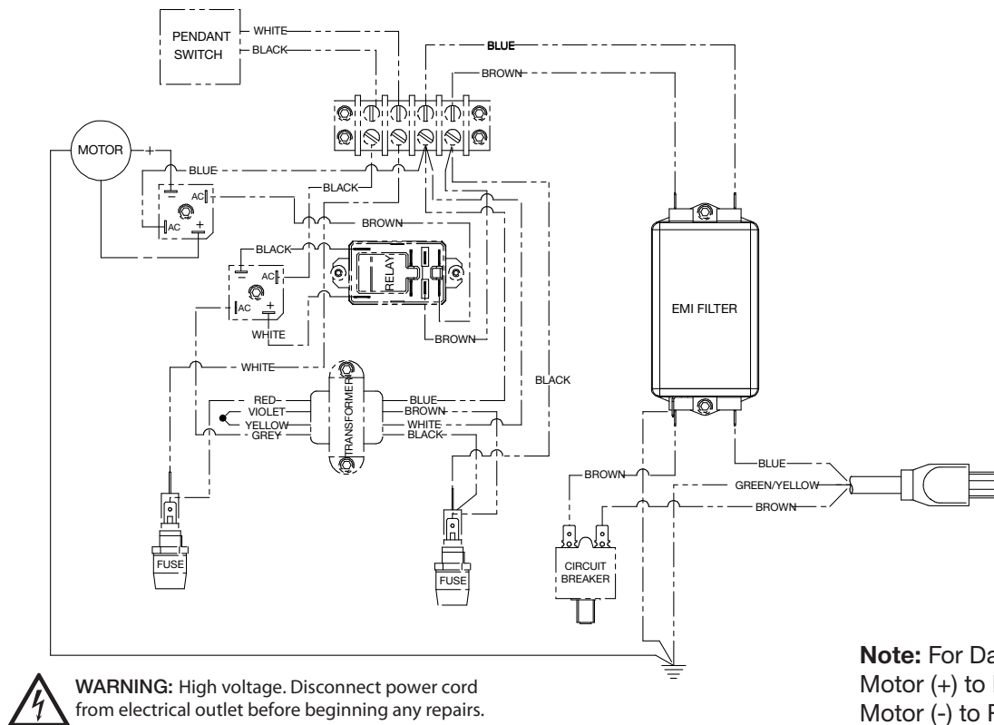
Figure 20 - 230 Volt Wiring Diagram
