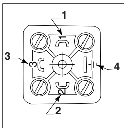
Abbildung 2, Elektrische Verbindung 1. Bezugspotential 2. Öffnerkontakt 3. Schließerkontakt 4. Masse
