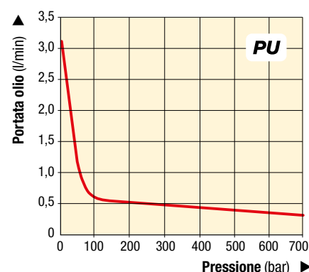
DIAGRAMMA DI PORTATA
