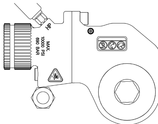
Fig 4.4-5 Sekskant muttertrekkersett reaksjon (Ingen reaksjonsarm) (Strammeposisisjon for RH gjenger)
