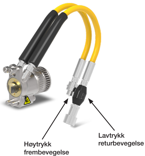
c. QD for muttertrekkerslange med skrukupling og sikkerhetsventil
