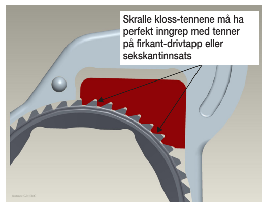
Fig 5.4-2 Inspeksjon skralle kloss
