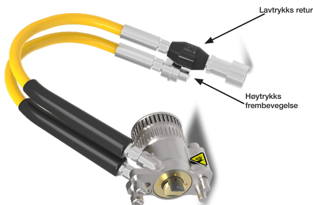
Fig 4.6-3 Muttertrekkerporter
