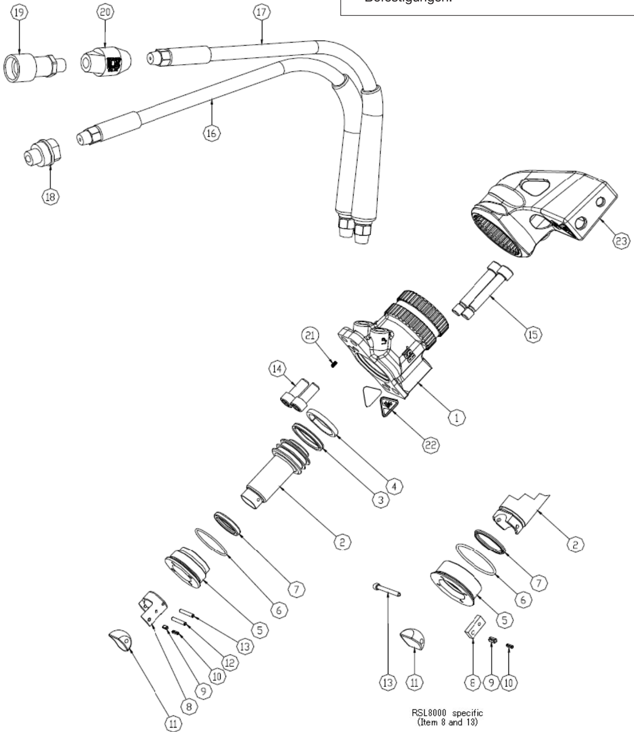
Abbildung 1, RSL-Drehmomentschlüsselantriebseinheit
