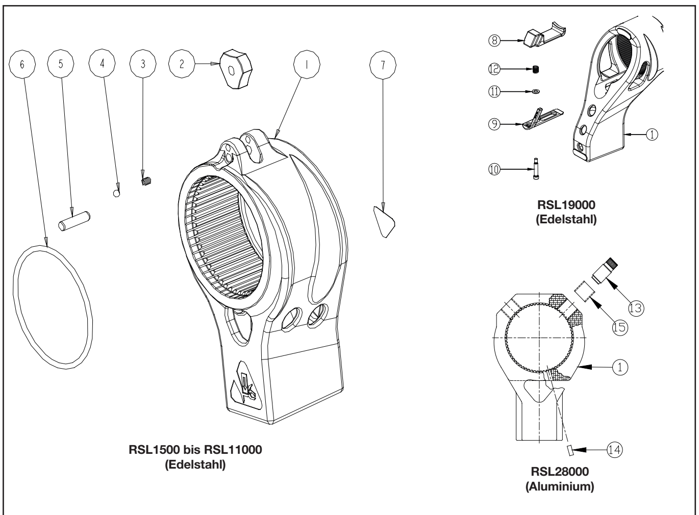
Abbildung 4, RSL-Abstützarmeinheit
