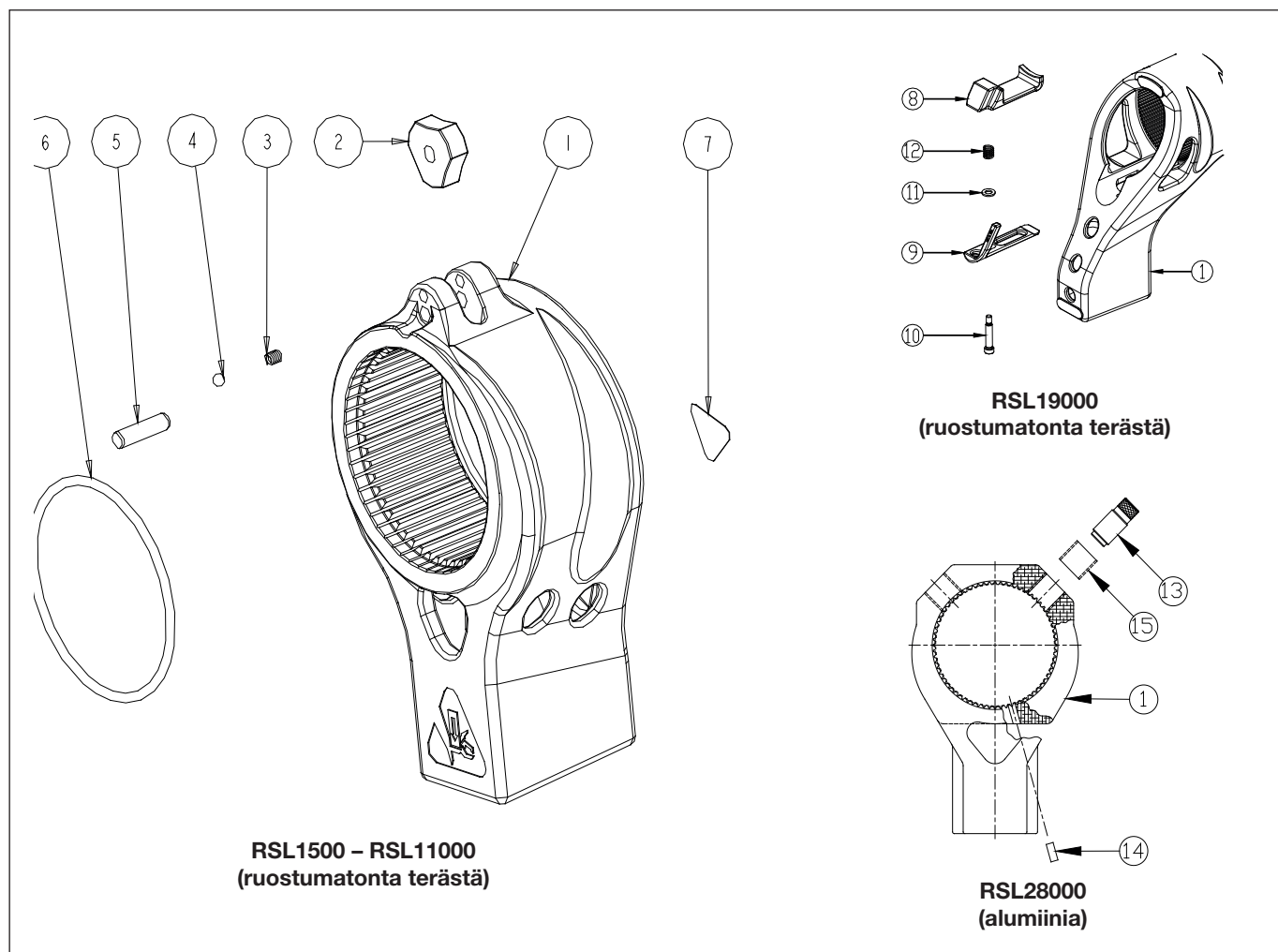
Kuva 4, RSL-tukivarsikokoonpano
