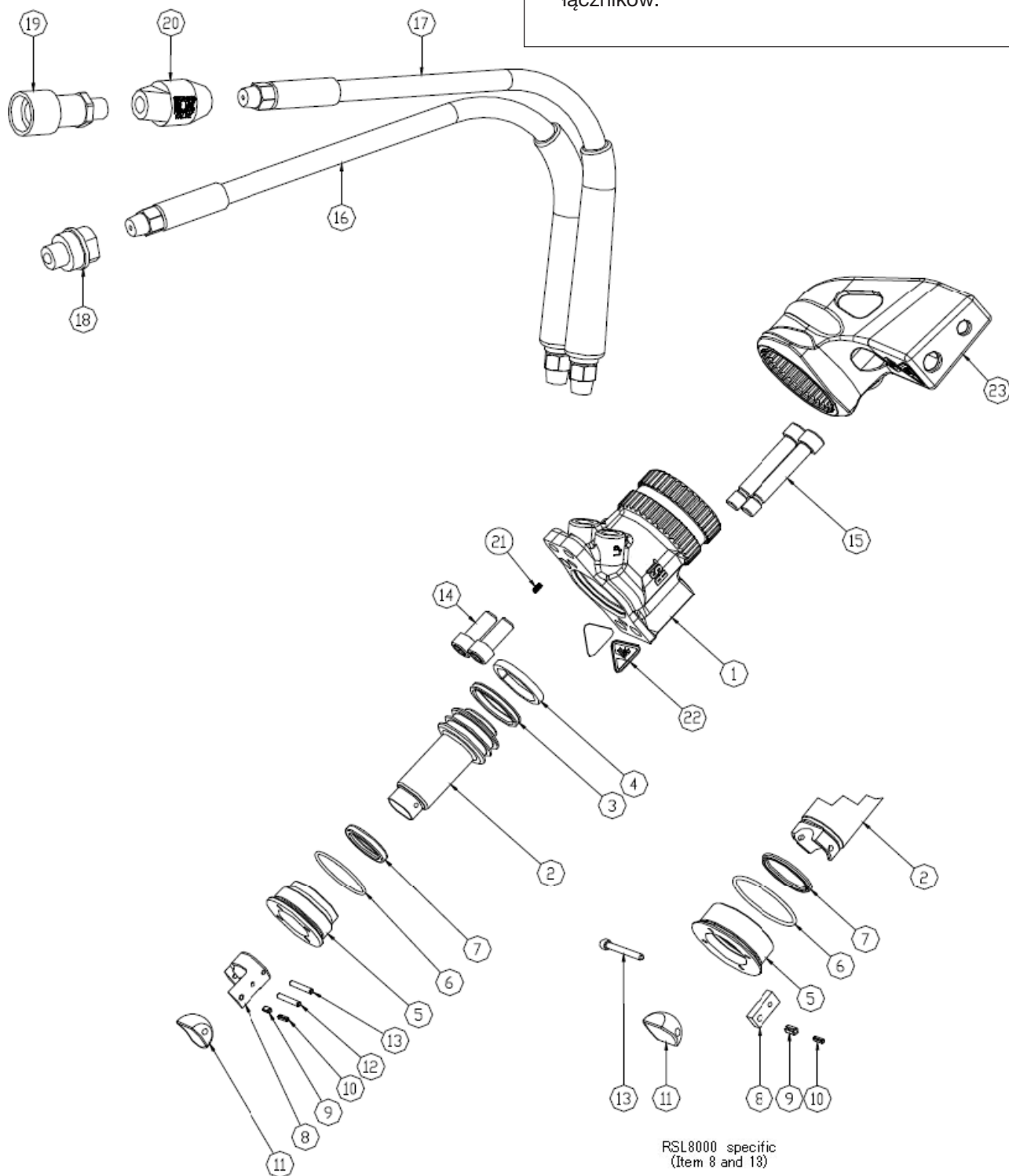
Rycina 1, Zespół klucza dynamometrycznego RSL
