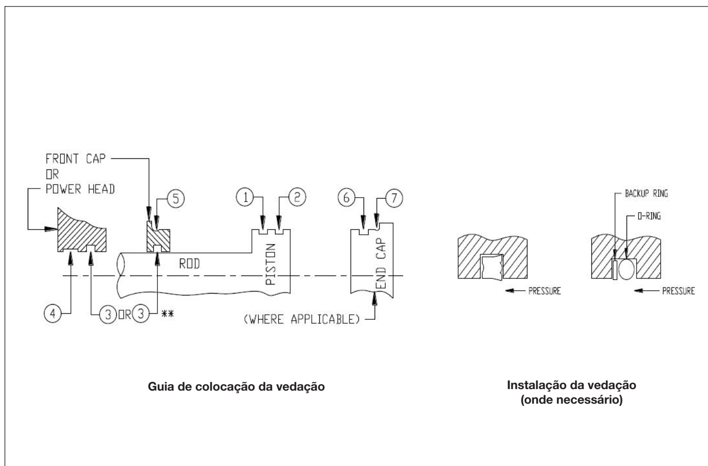
Figura 5, conjunto de vedações para unidade de acionamento de chaves de torque RSL
