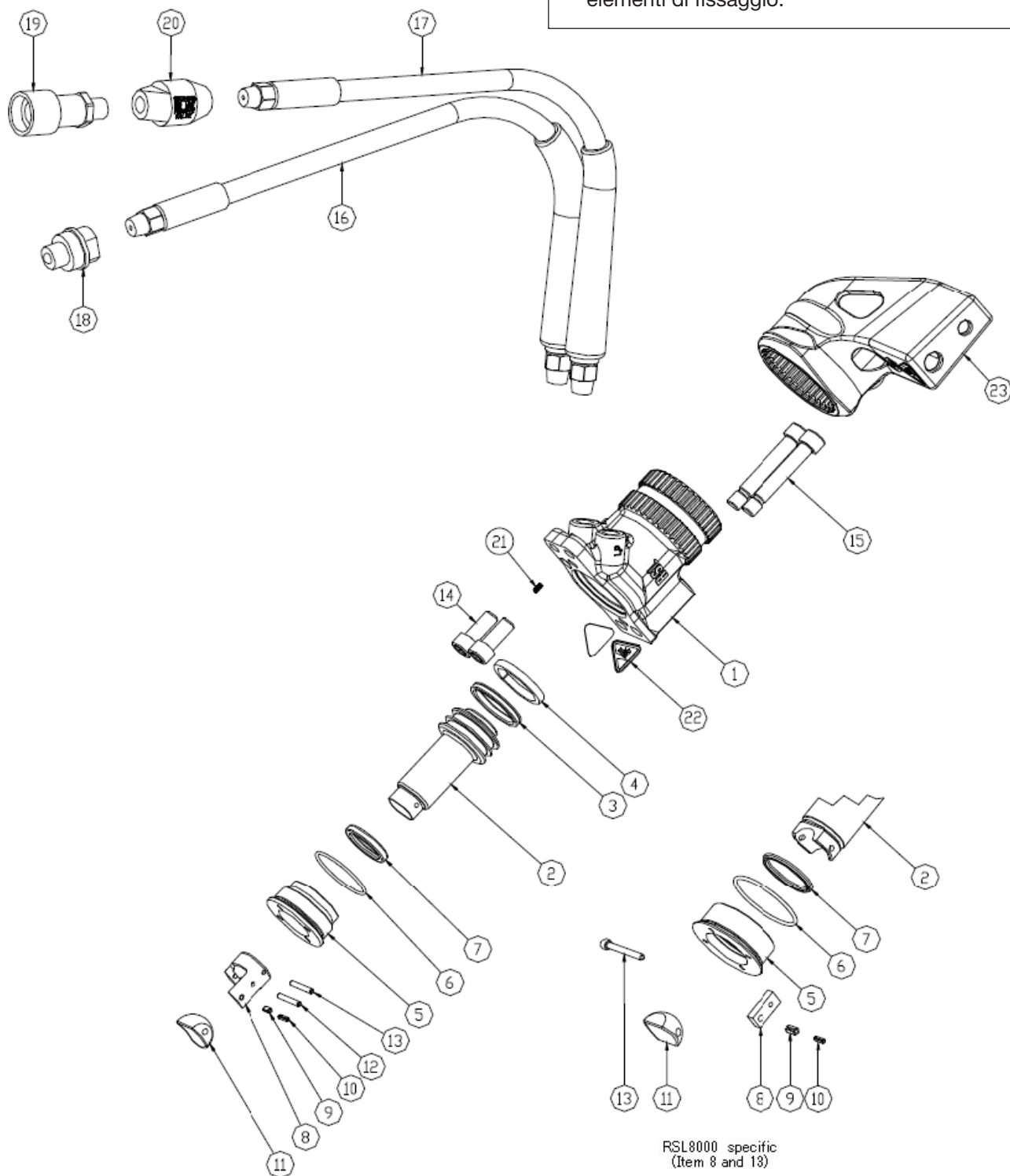
Figura 1, Assemblaggio unità di azionamento chiave RSL
