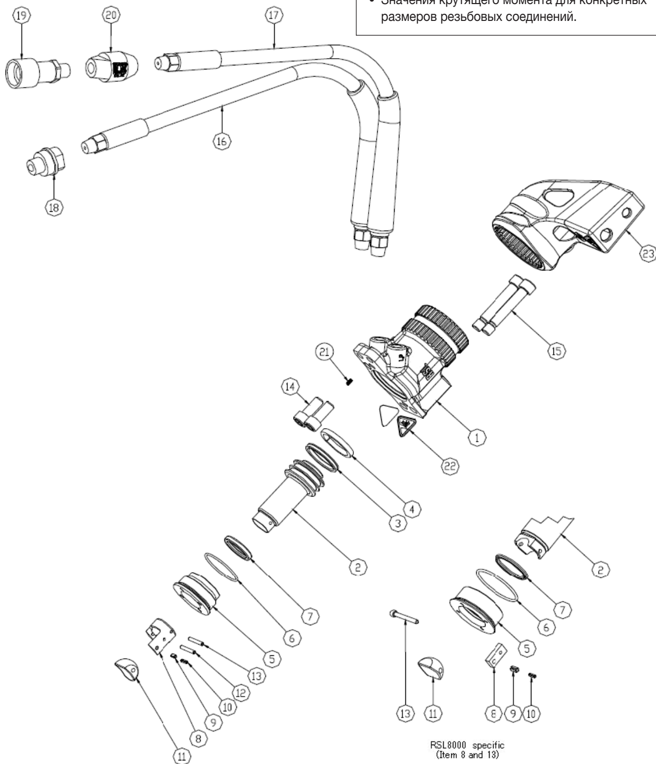
Рисунок 1. Узел привода для гидравлических гайковертов серии RSL
