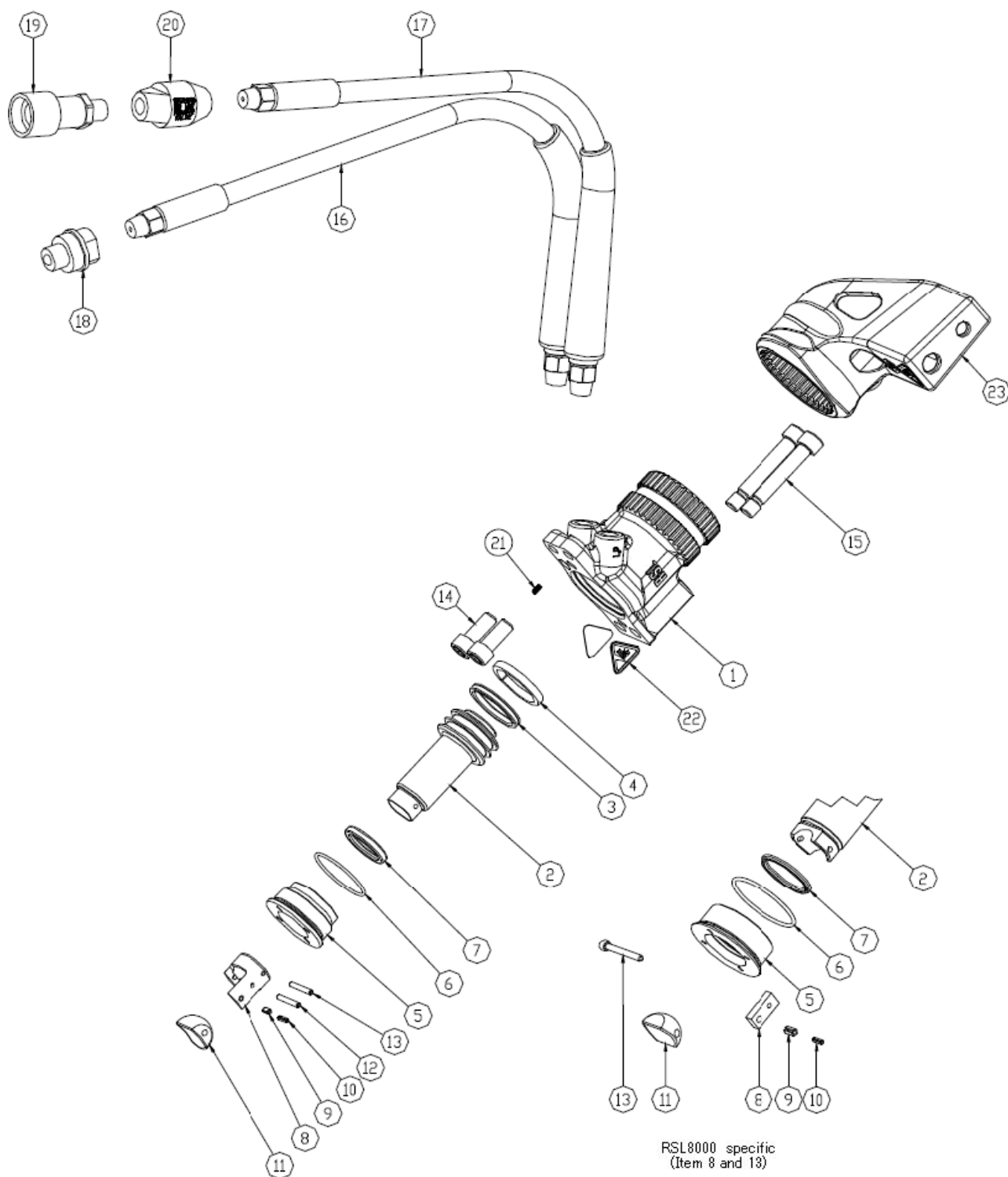
Figur 1, RSL-momentverktygets delar
