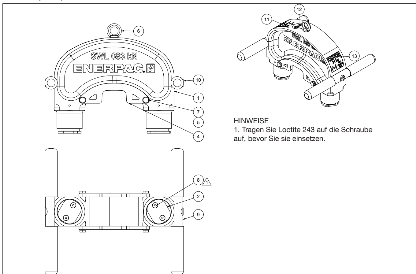
Abbildung 10: Hauptkomponenten Klemme
