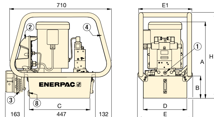
Serie ZE con depósito de 9,8 - 19,8 - 39 litros
