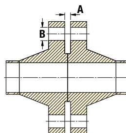
Dimensioni flangia
