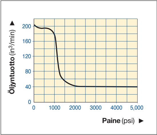
ZW2-SARJA (BRITTLÄINEN)
