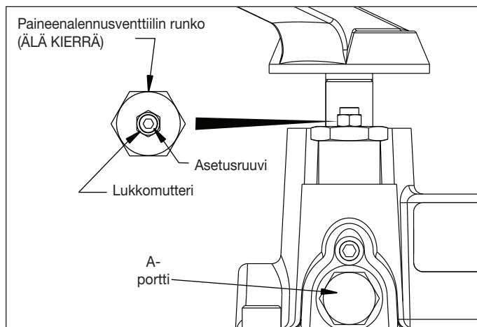
Kuva 15: Paineenalennusventtiili – VM32
