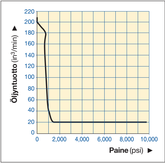
ZE2-SARJA (BRITTLÄINEN)
