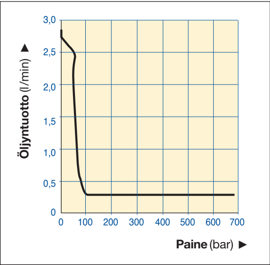
ZE2-SARJA (METRINEN)
