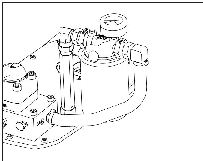
Rysunek 18: Filtr przewodu powrotnego oleju (opcjonalny)
