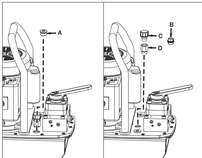
Rysunek 3: Umiejscowienie korków wlewu oleju oraz odpowietrznika zbiornika
