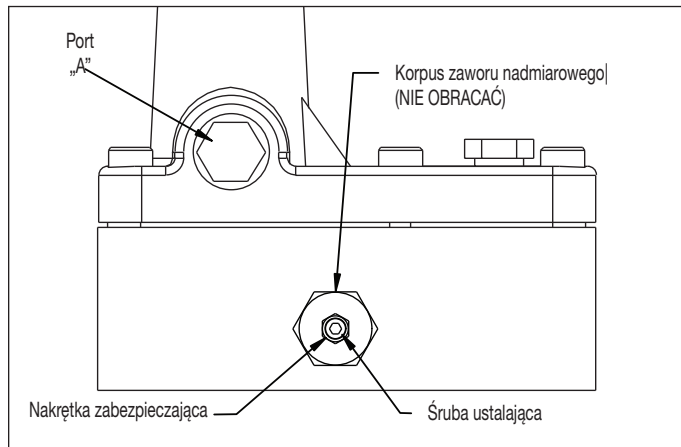
Rysunek 14: Zawór nadmiarowy – VM22
