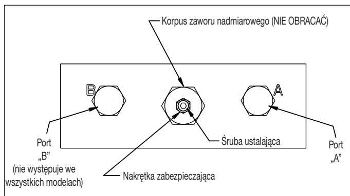
Rysunek 16: Zawór nadmiarowy – serie VM, VE i VEW33 & 43
