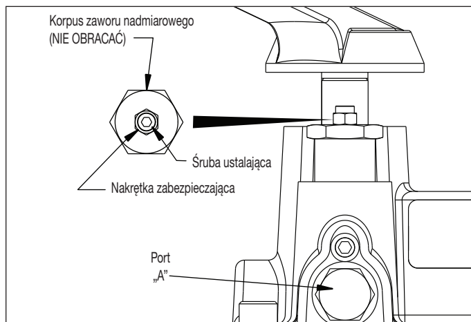
Rysunek 15: Zawór nadmiarowy – VM32
