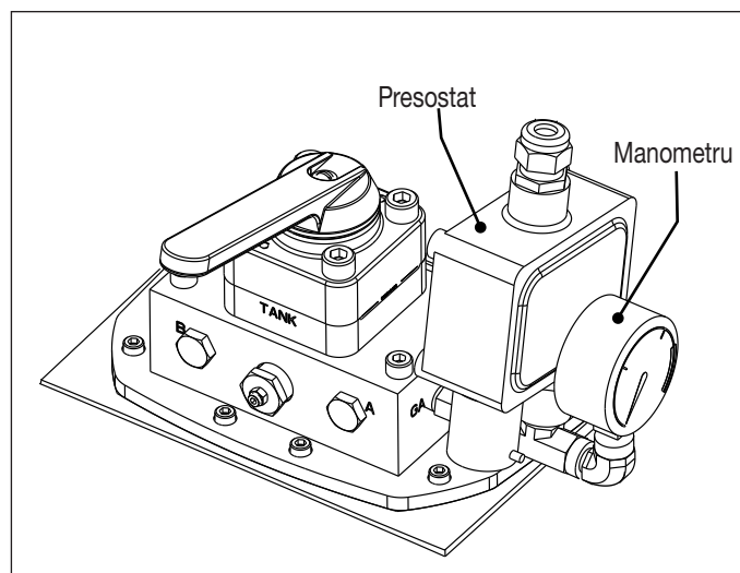
Figura 11: Presostatul și manometrul
