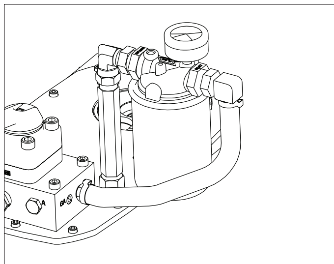
Figur 18: Returledningsoljefilter (F)
