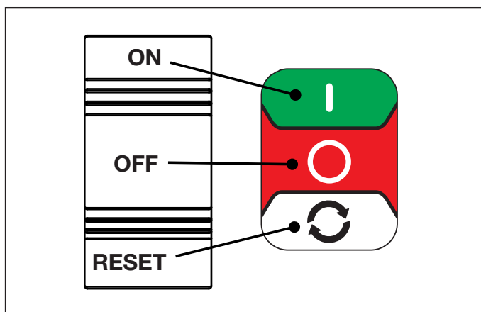
Figur 6: Vippströmbrytare
