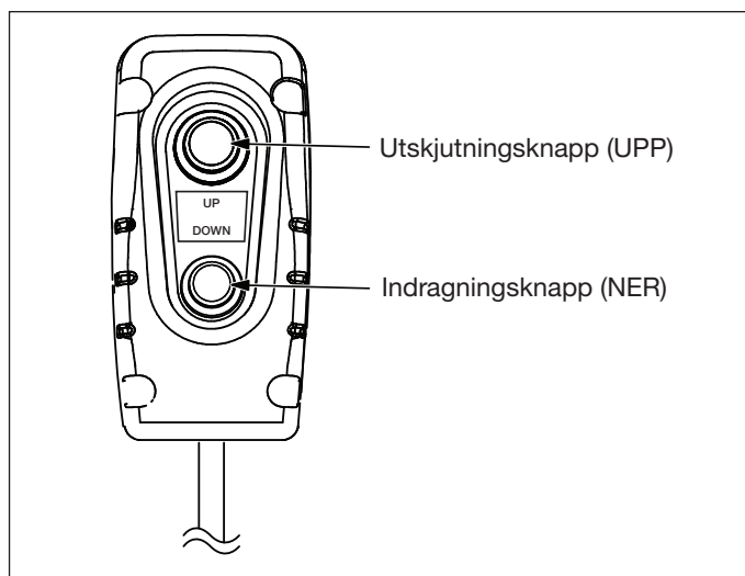
Figur 10: Manöverdosa med två knappar
