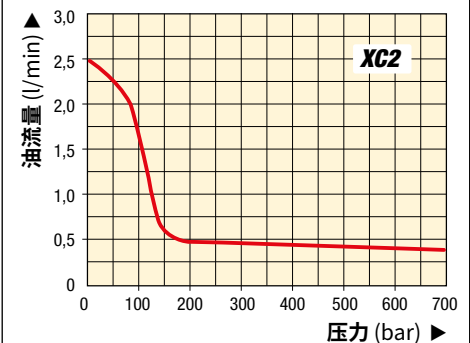
油流量VS压力
