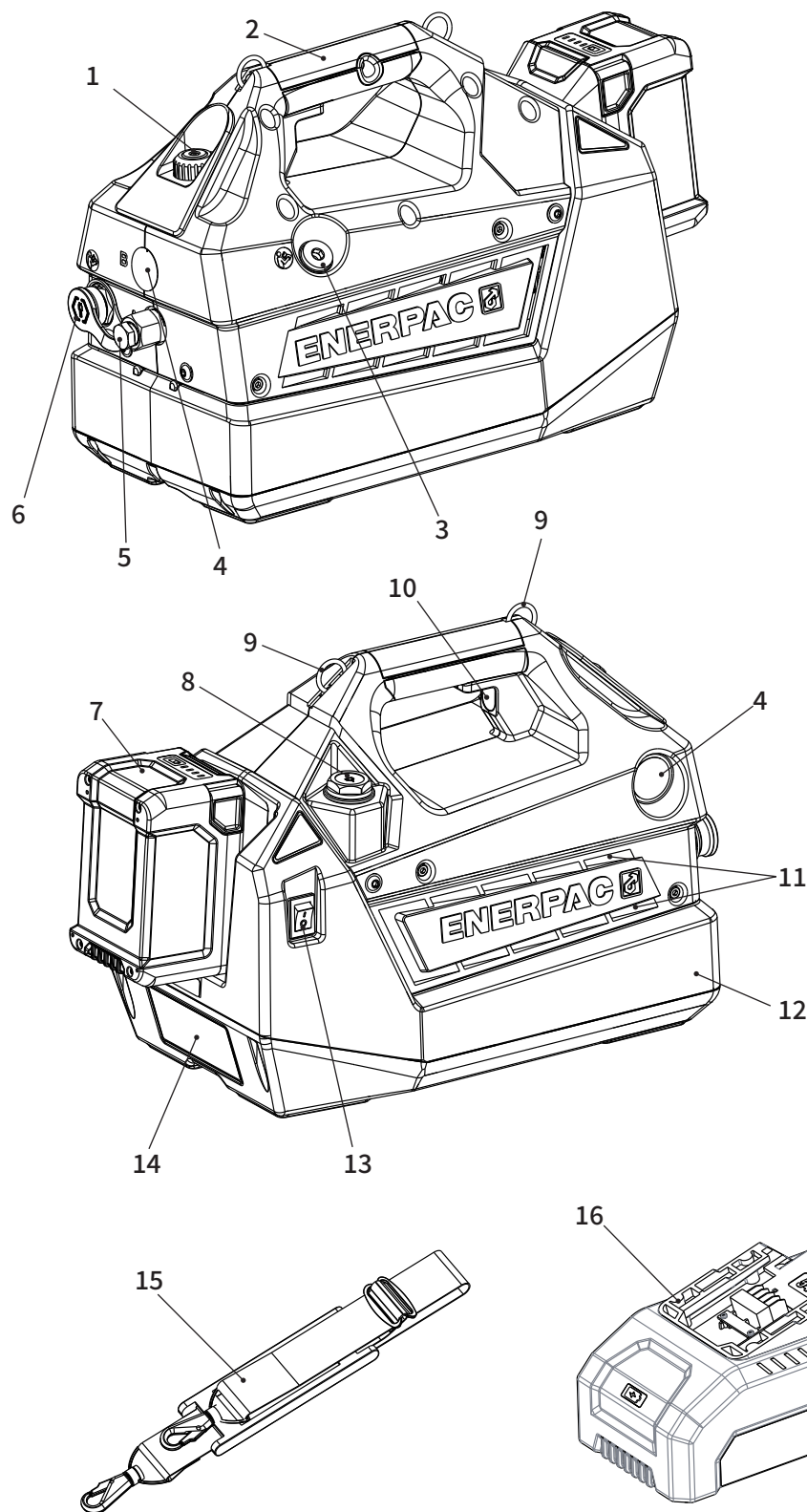
図1: 特長と構成部品、モデルXC2302SおよびXC2304S
