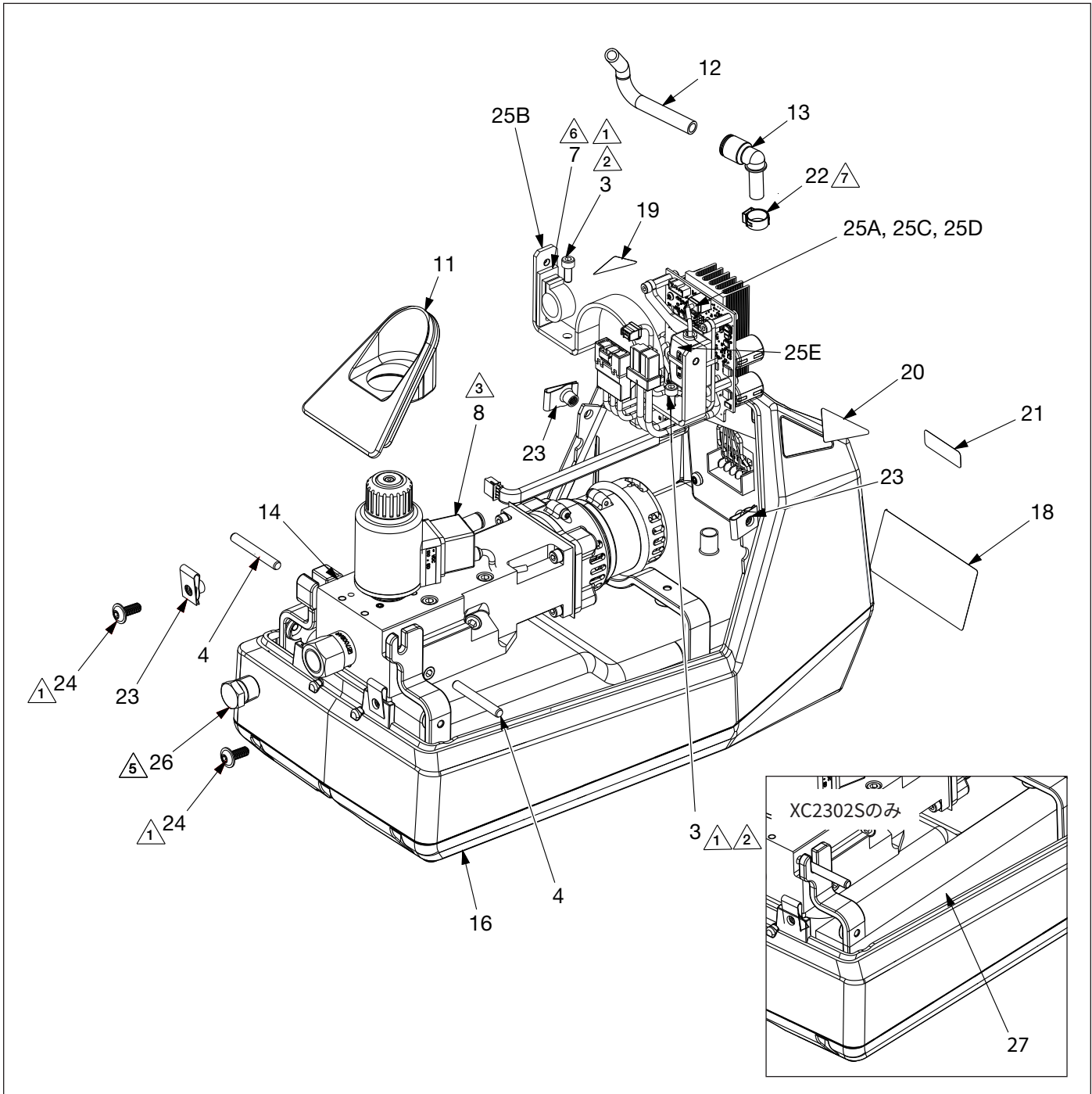
図16: メインアセンブリ
