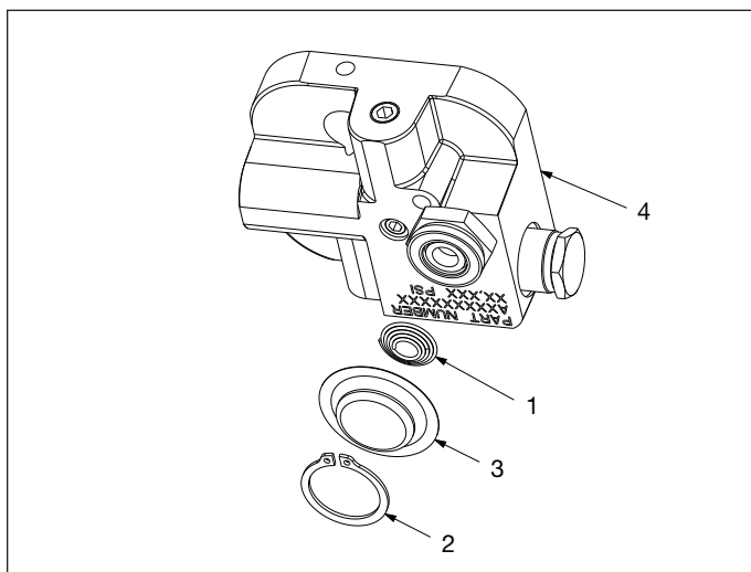
図24: ポンプエレメント
