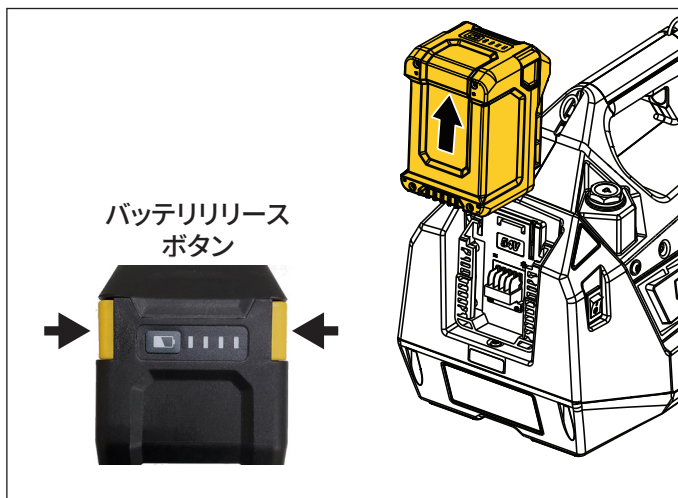
図8: バッテリー - 取り外し
