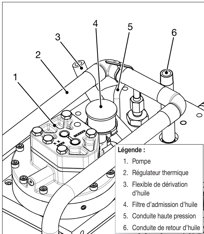
Figure 19 : inspection et nettoyage - pompe
