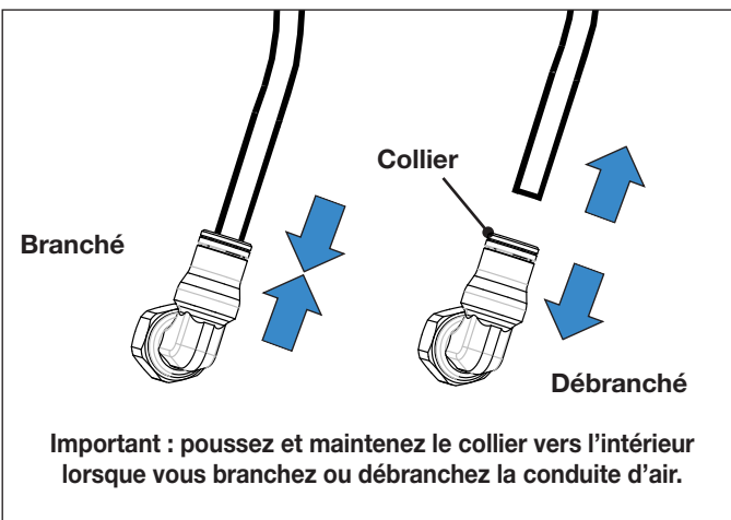
Figure 12 : Raccordement des conduites d'air
