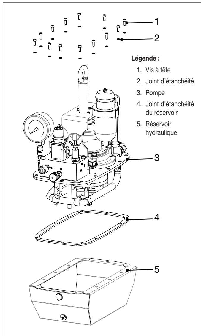
Figure 18 : Pompe et réservoir hydraulique
