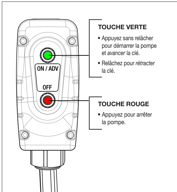
Figure 8 : Démarrage et arrêt de la pompe
