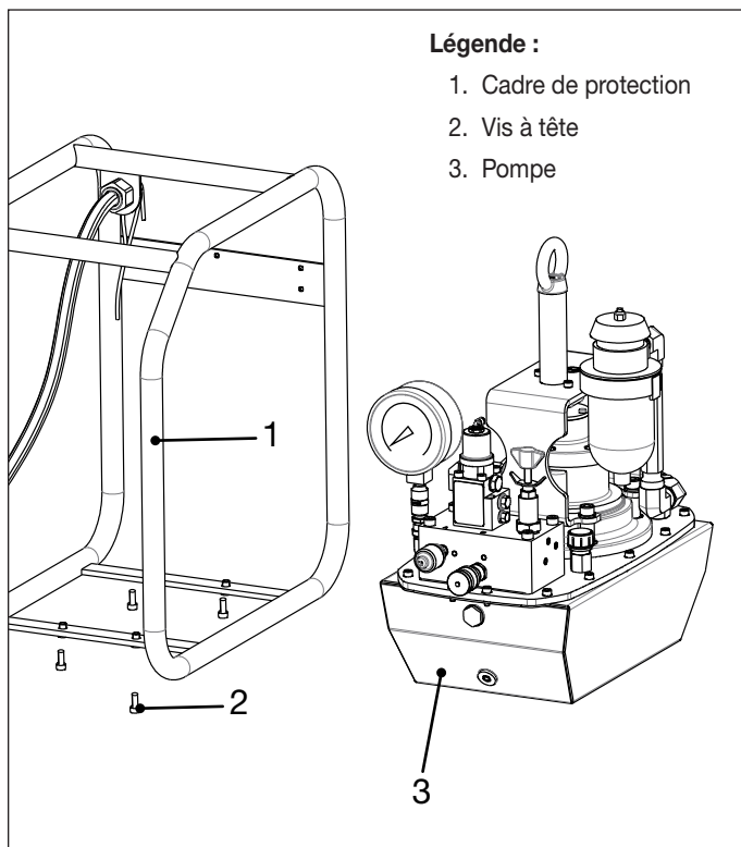
Figure 17 : Pompe et cadre de protection
