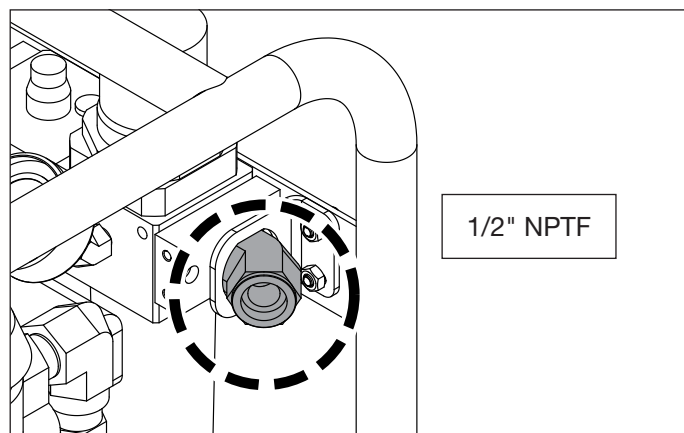
Figure 5 : Raccordement du circuit d'air comprimé (entrée d'air)
