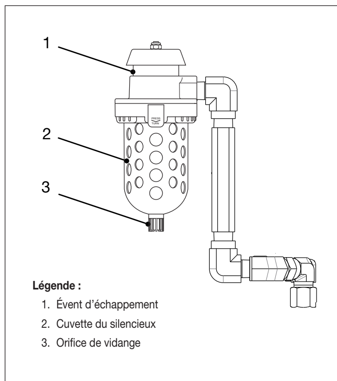
Figure 20 : Silencieux d'échappement pneumatique
