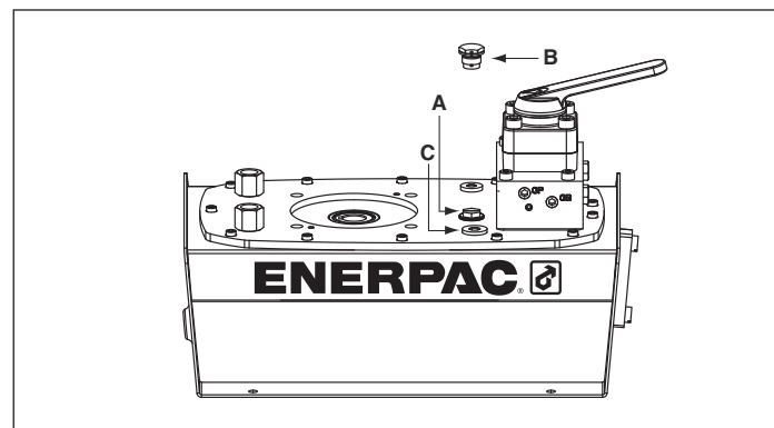
Figuur 2, ZG Ontluchtingsinstallatie
