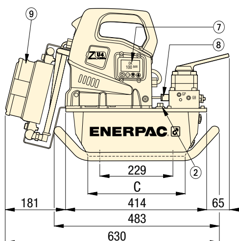
Serie ZU4 con depósitos de 4,6 y 6,8 litros
