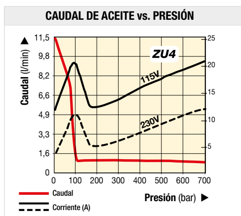
SERIE ZU4 TABLA DE RENDIMIENTO
