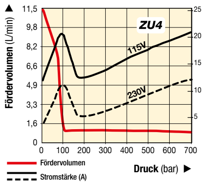
FÖRDERDIAGRAMM
